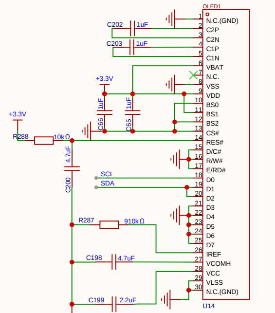
OLED-SSD1315
