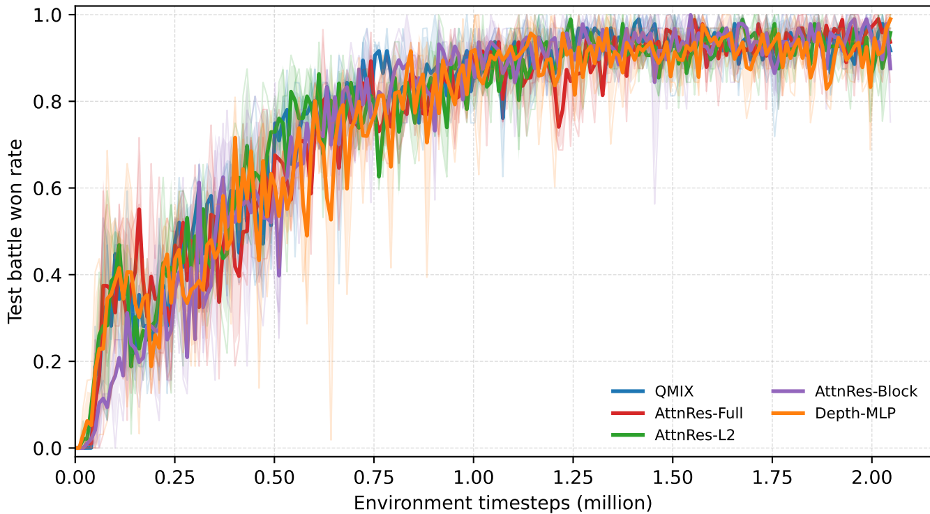
3s5z: QMIX Variants
