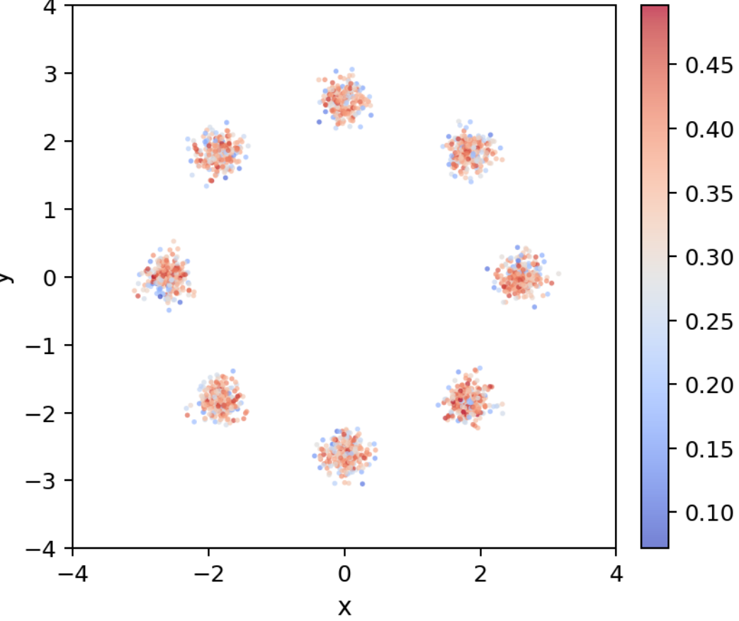
Local Curvature
