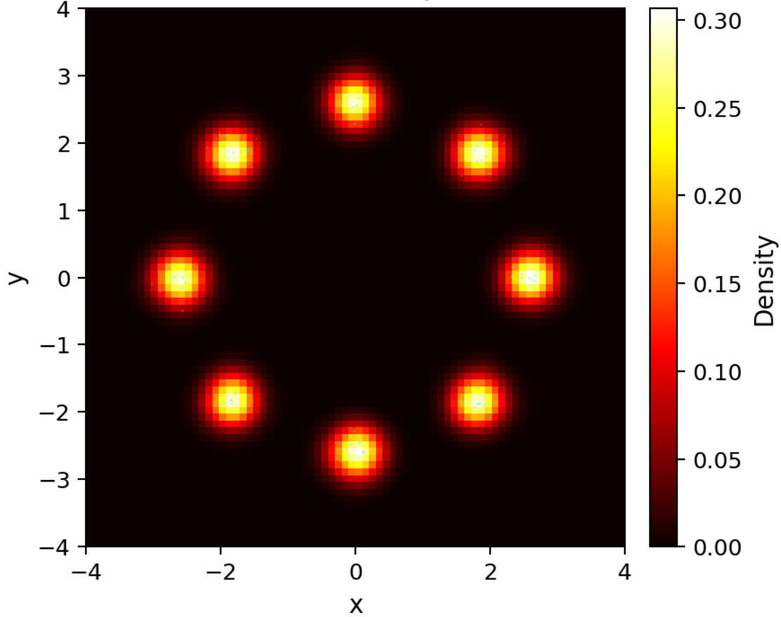
KDE Density
