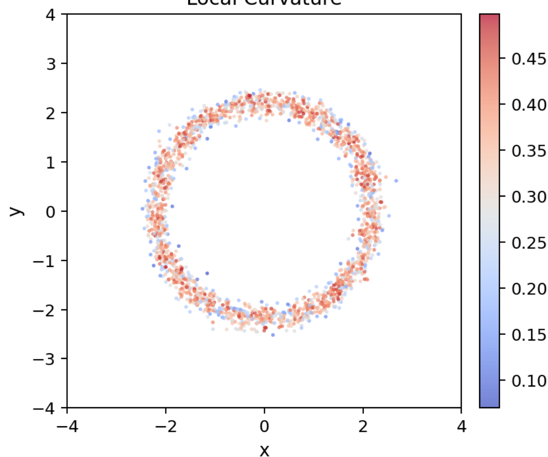
Local Curvature
