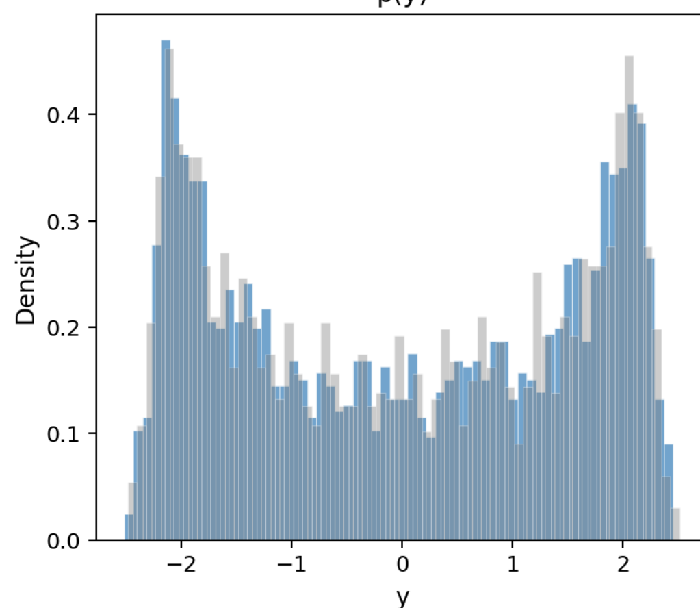
p(y)
