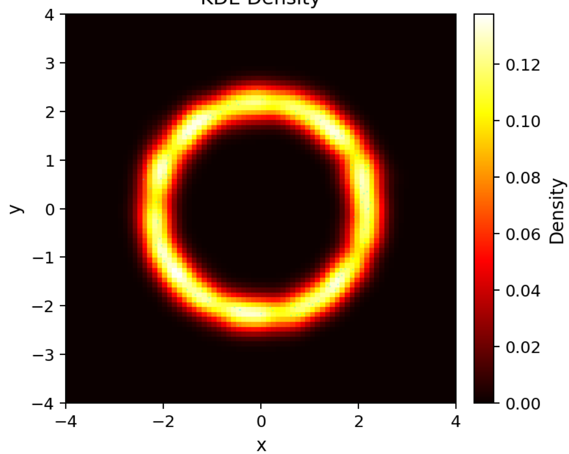
KDE Density
