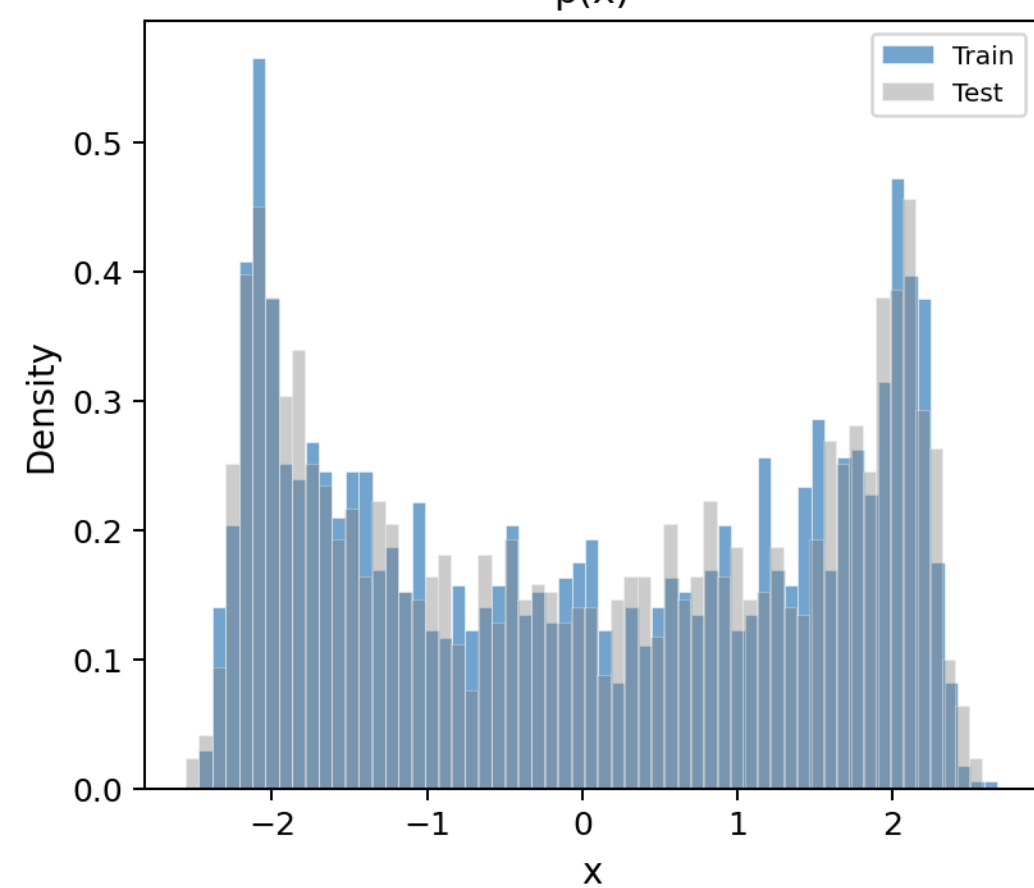
p(x)
