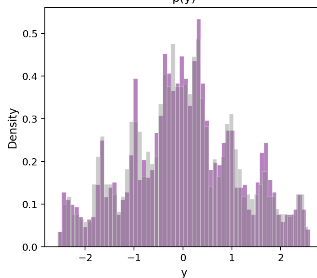
p(y)
