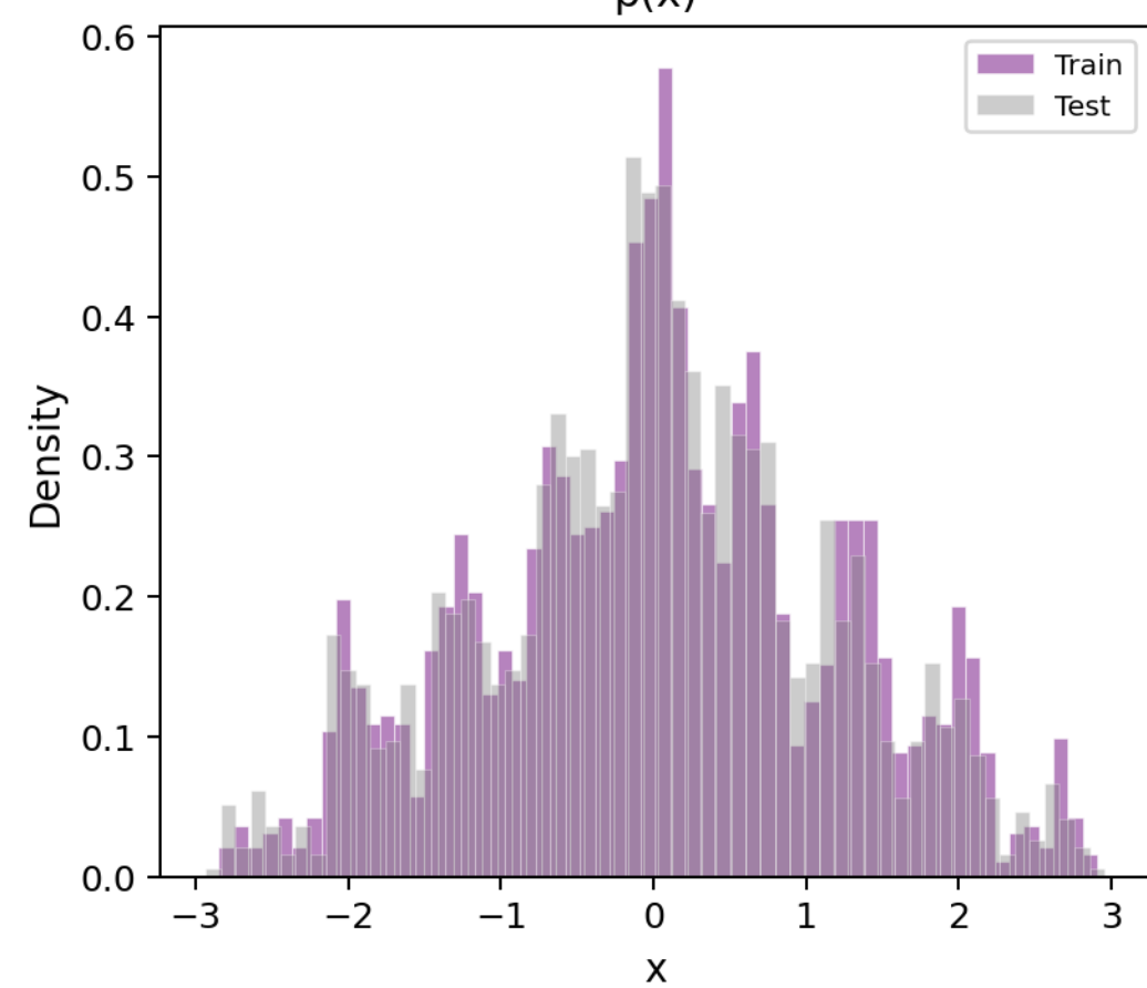
p(x)
