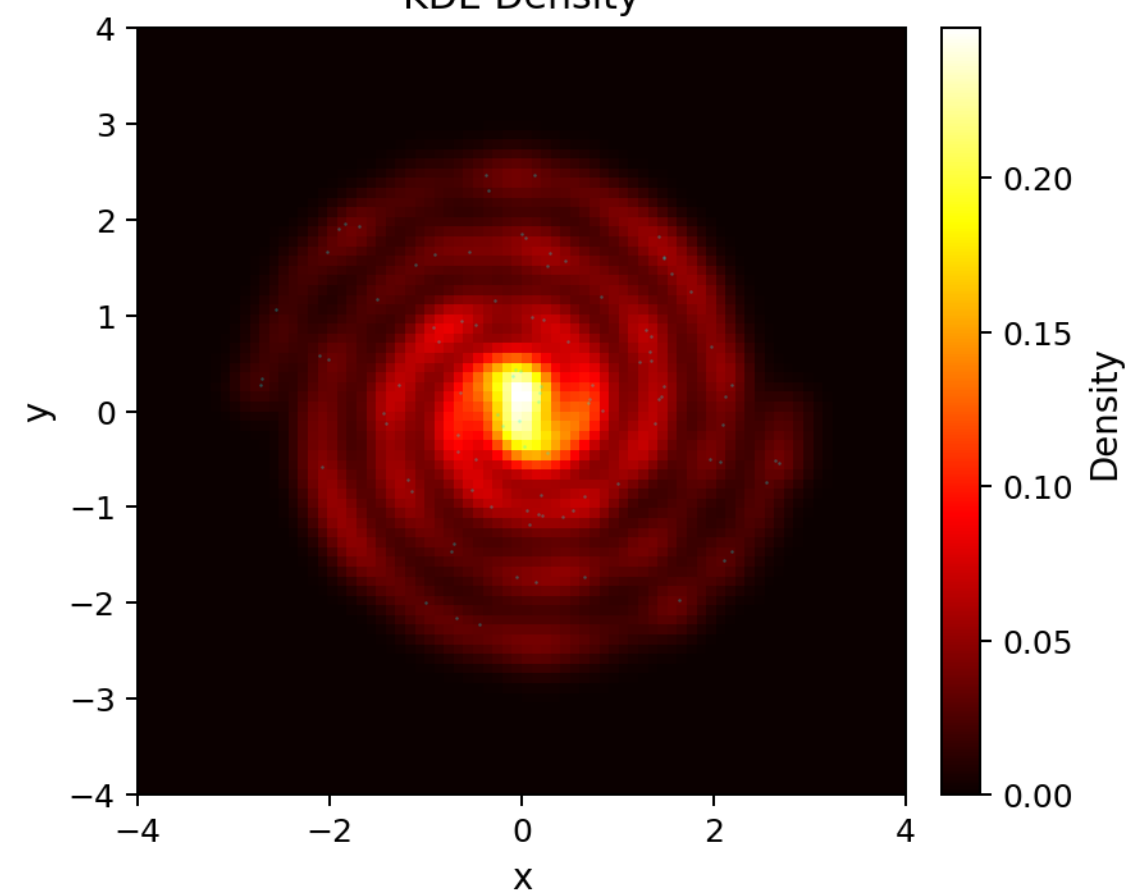
KDE Density
