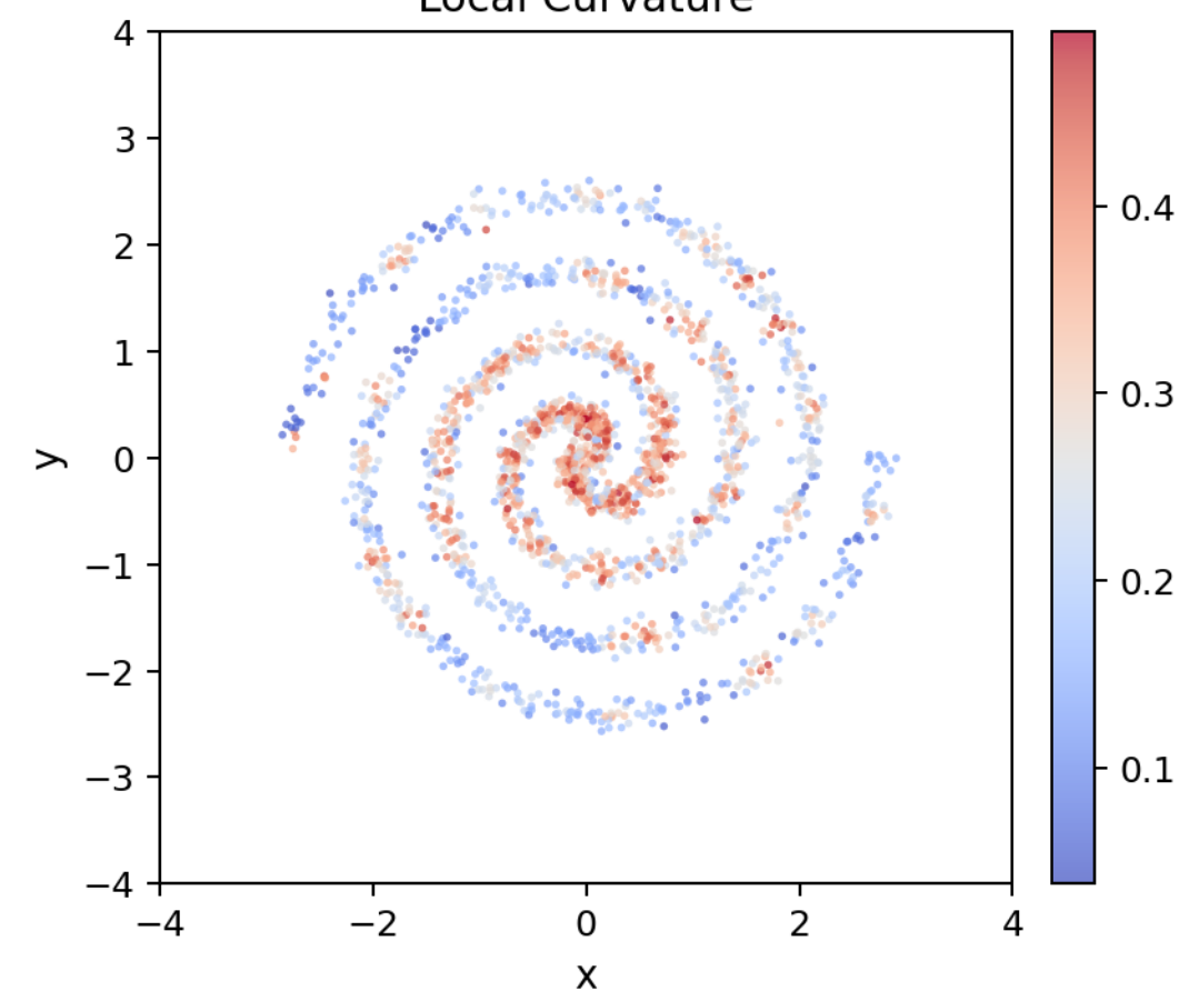
Local Curvature
