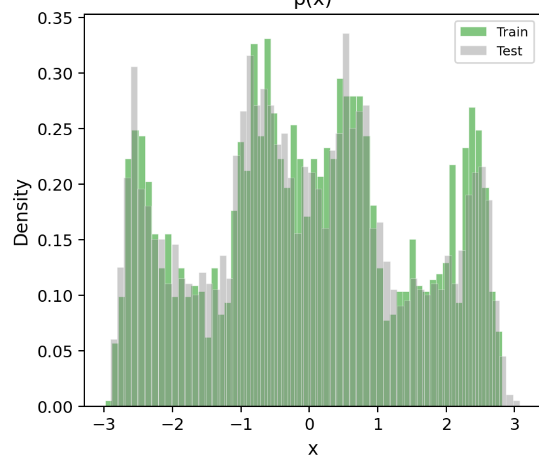
p(x)
