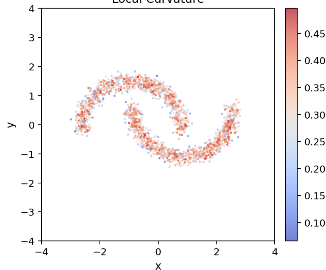
Local Curvature
