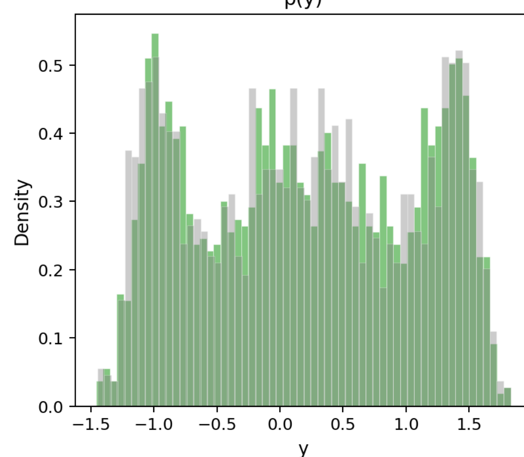
p(y)
