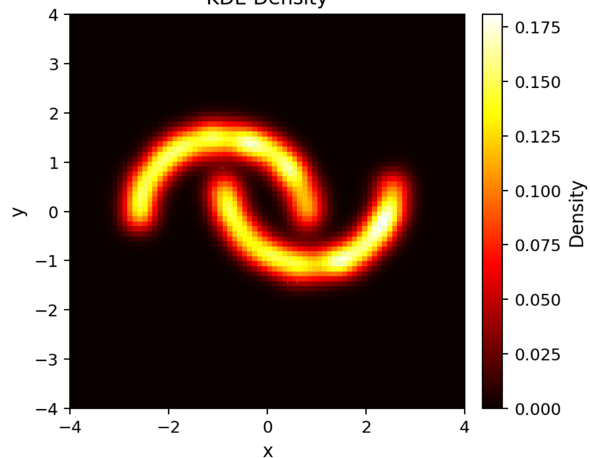
KDE Density
