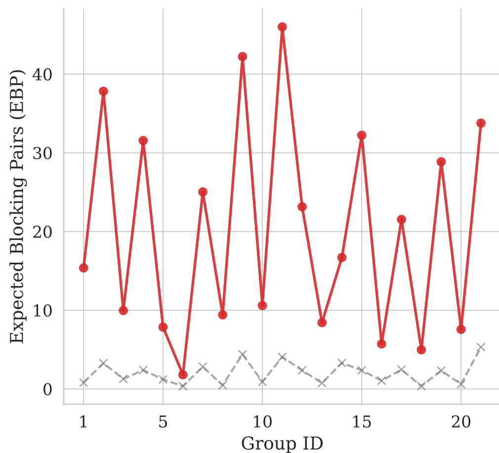
(d) Gemini-Flash
