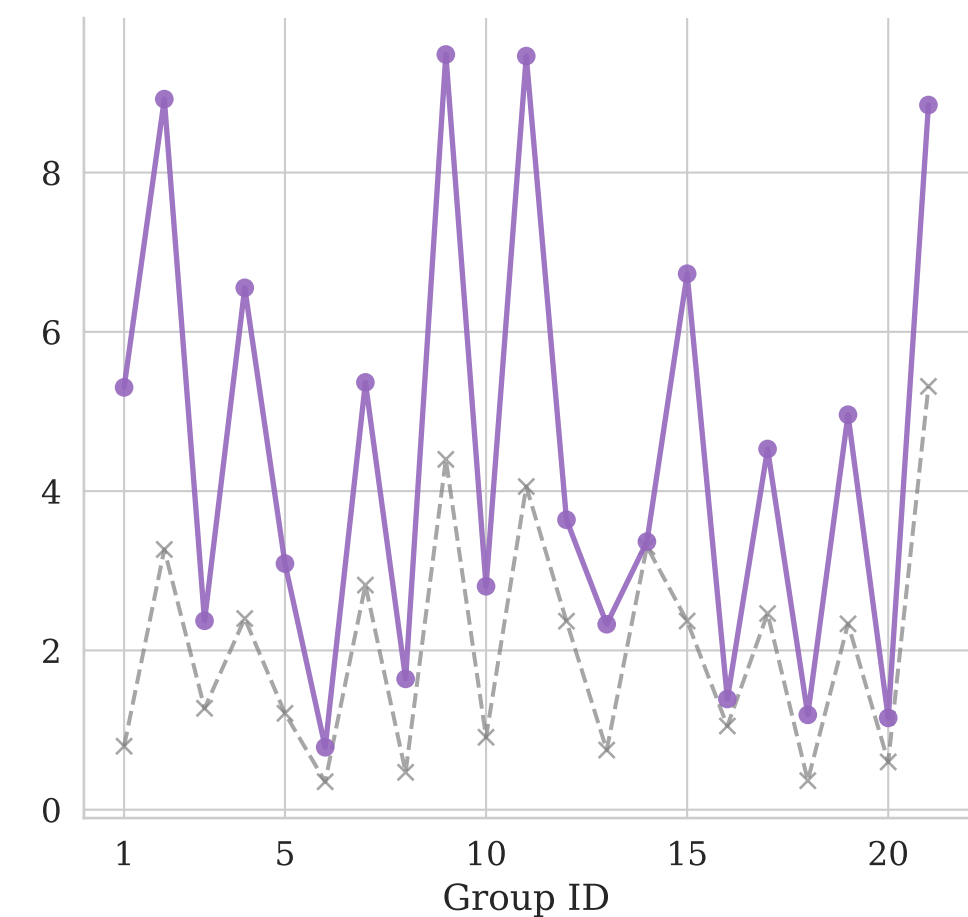
(e) Qwen-72B
