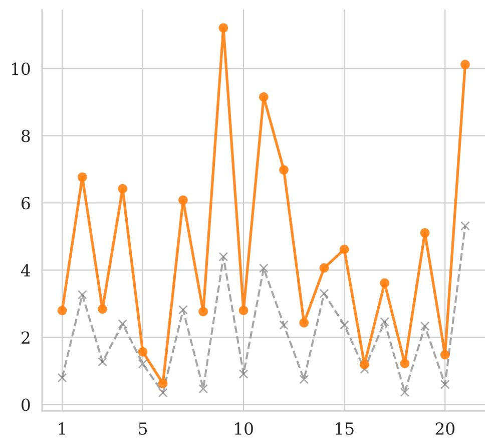
(b) Claude-Sonnet
