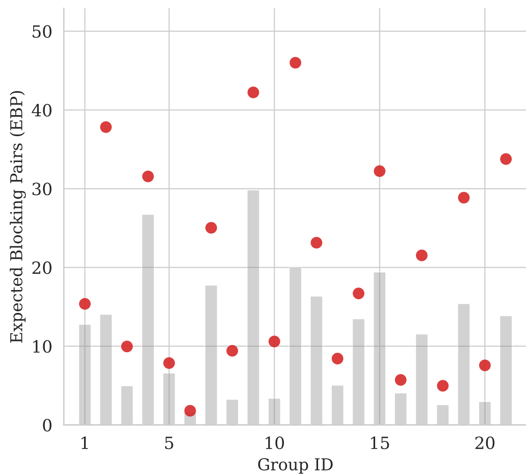
(d) Gemini-Flash
