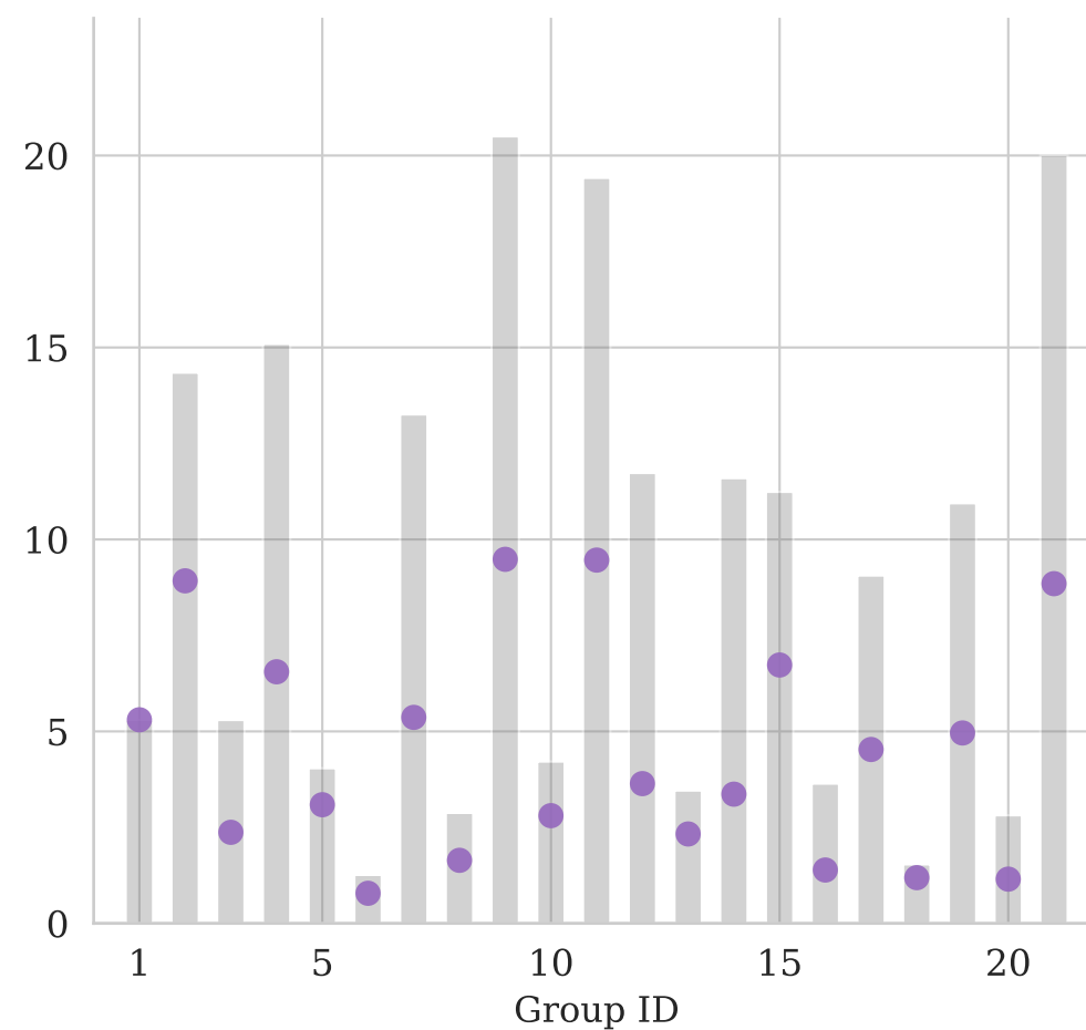
(e) Qwen-72B
