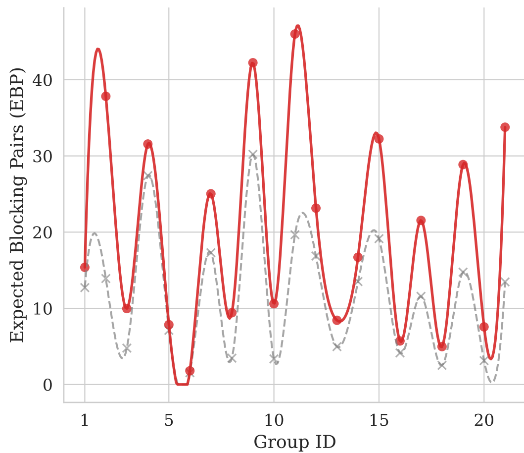
(d) Gemini-Flash
