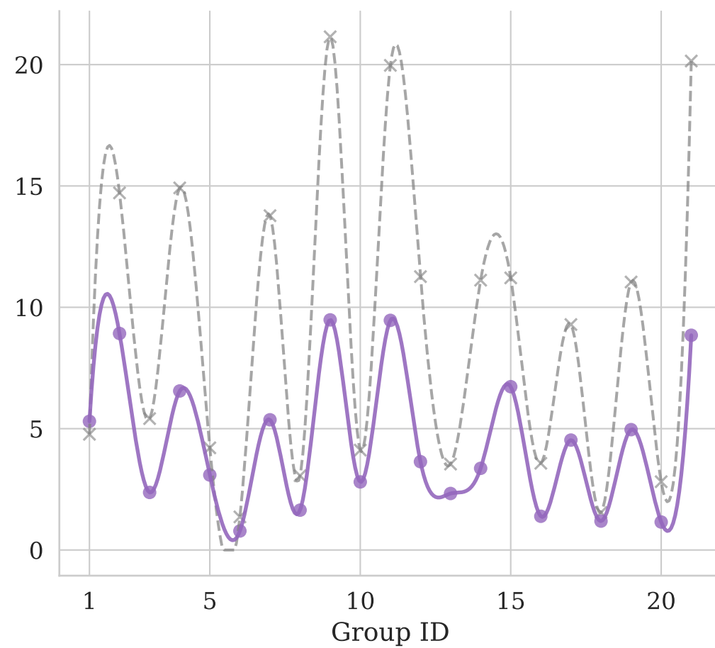
(e) Qwen-72B
