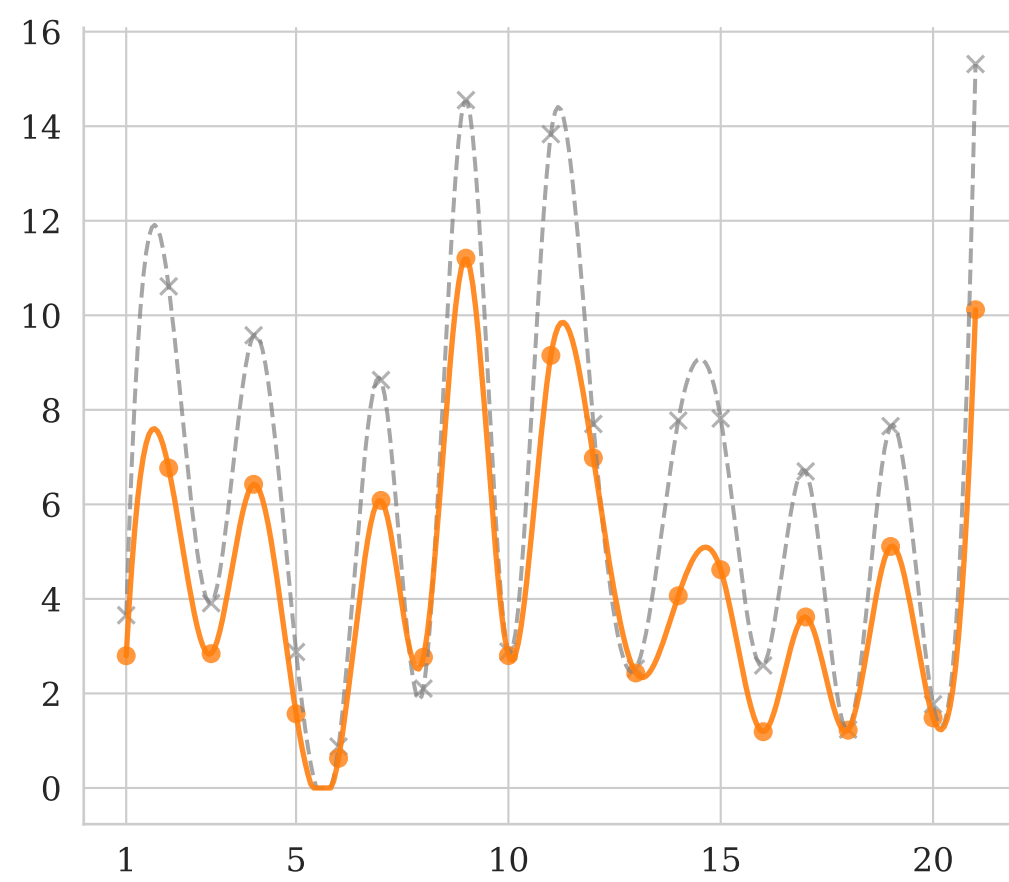
(b) Claude-Sonnet
