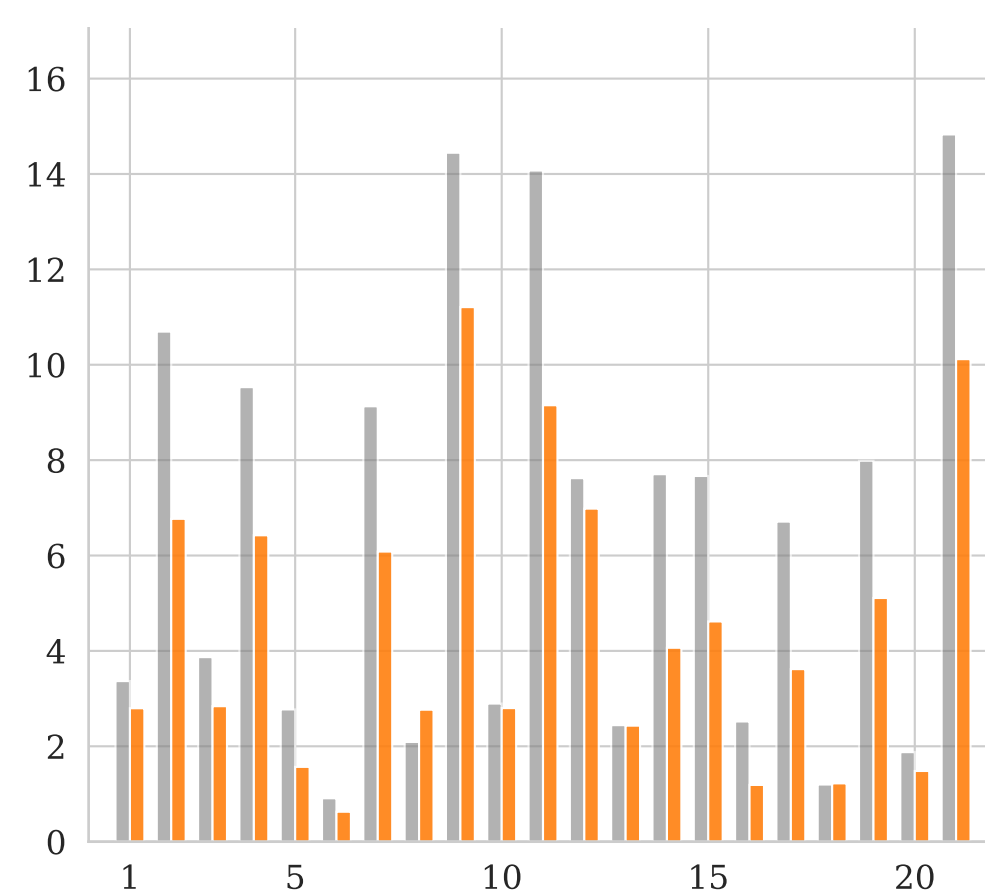
(b) Claude-Sonnet
