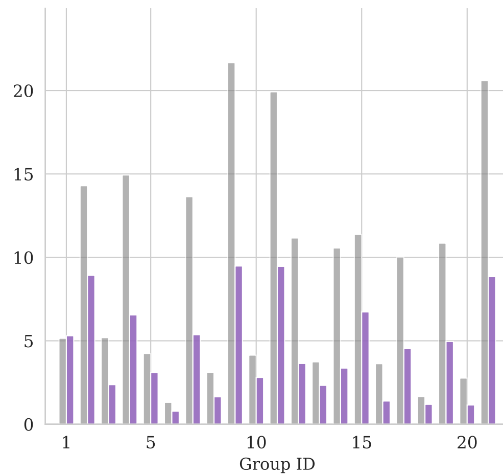
(e) Qwen-72B
