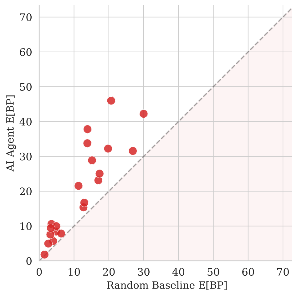
(d) Gemini-Flash
