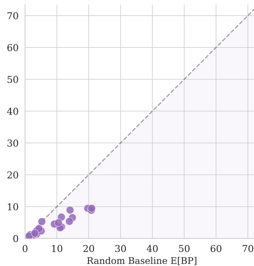
(e) Qwen-72B
