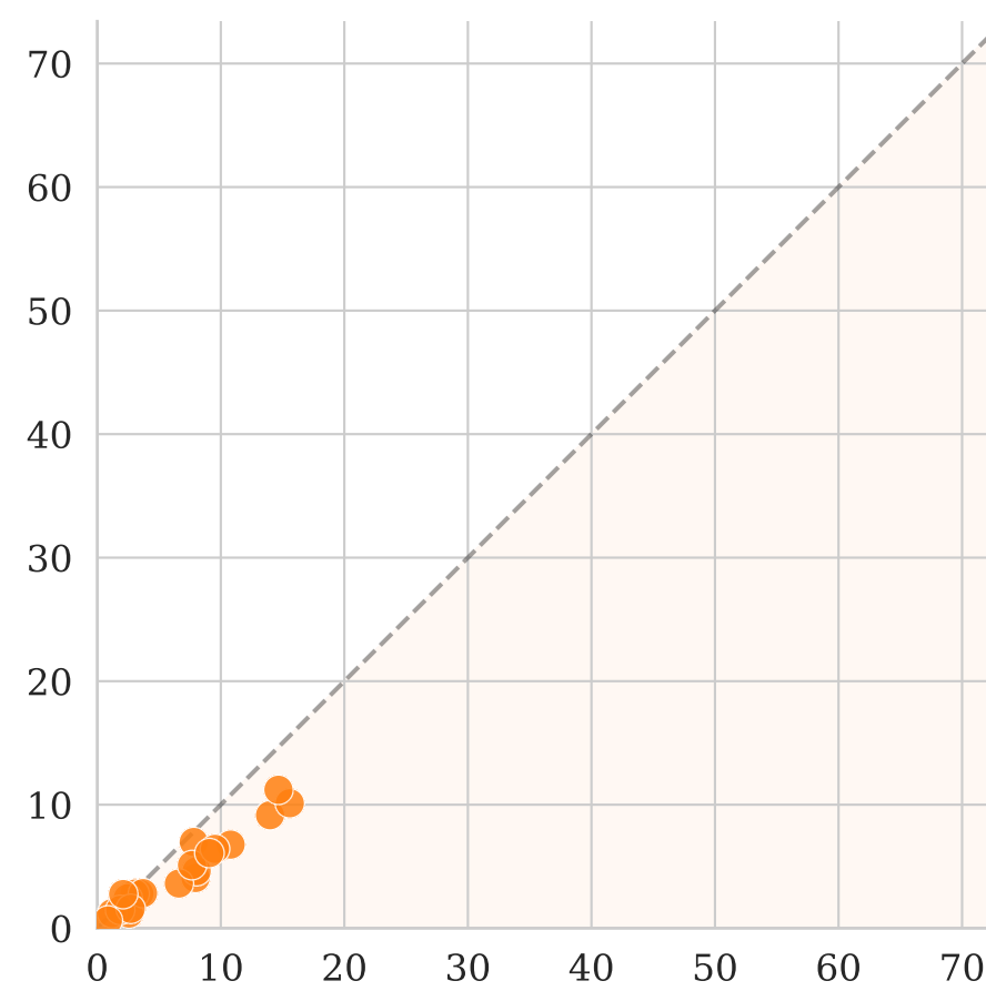
(b) Claude-Sonnet
