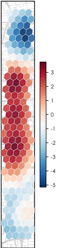
Gi* life hotspot (Hot 48 · Cold 36 · NS 67)
