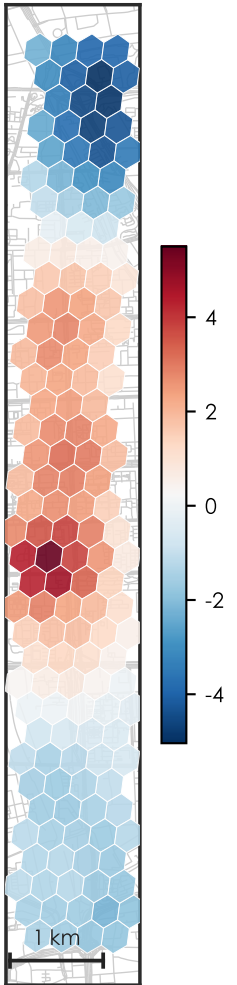
Gi* industry hotspot (Hot 37 · Cold 24 · NS 90)
