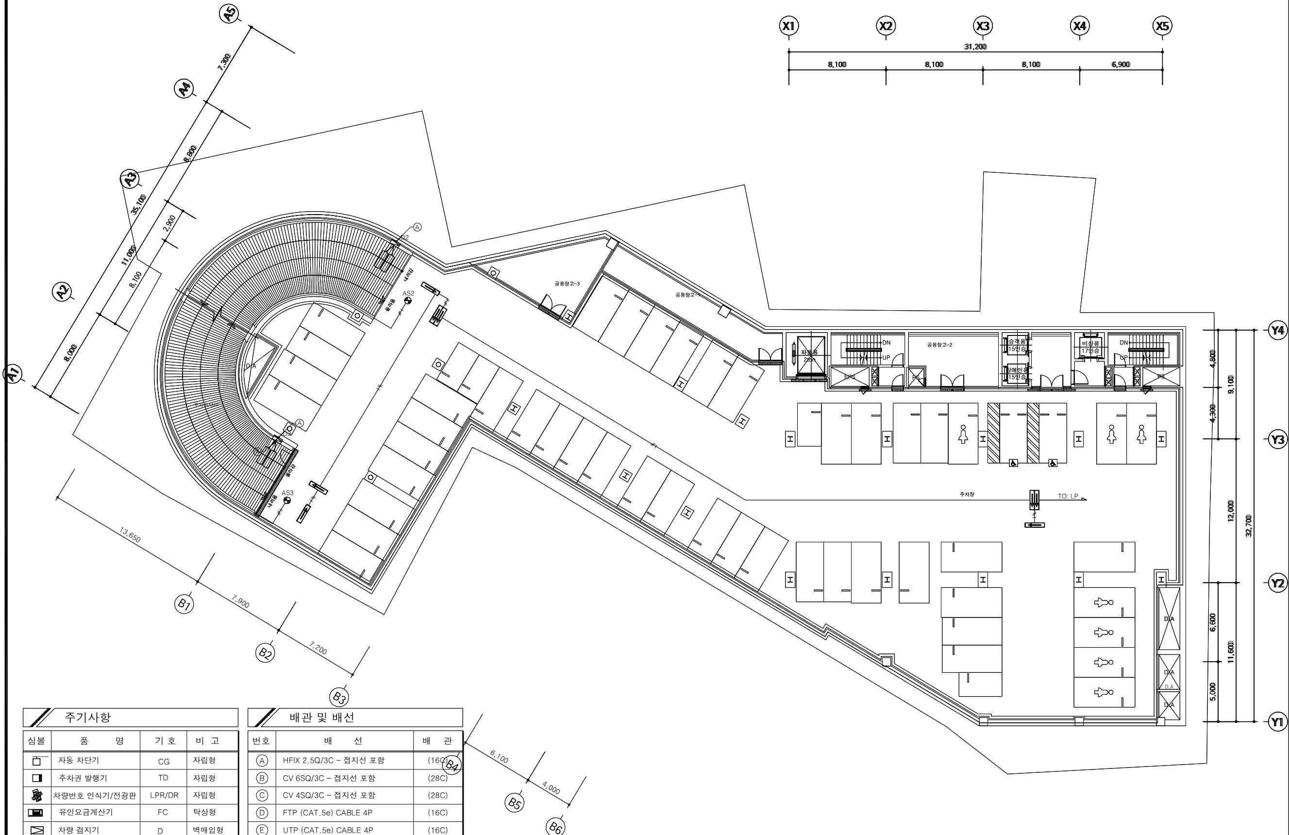
지하 3층 주차관제설비 평면도 SCALE:1/150
