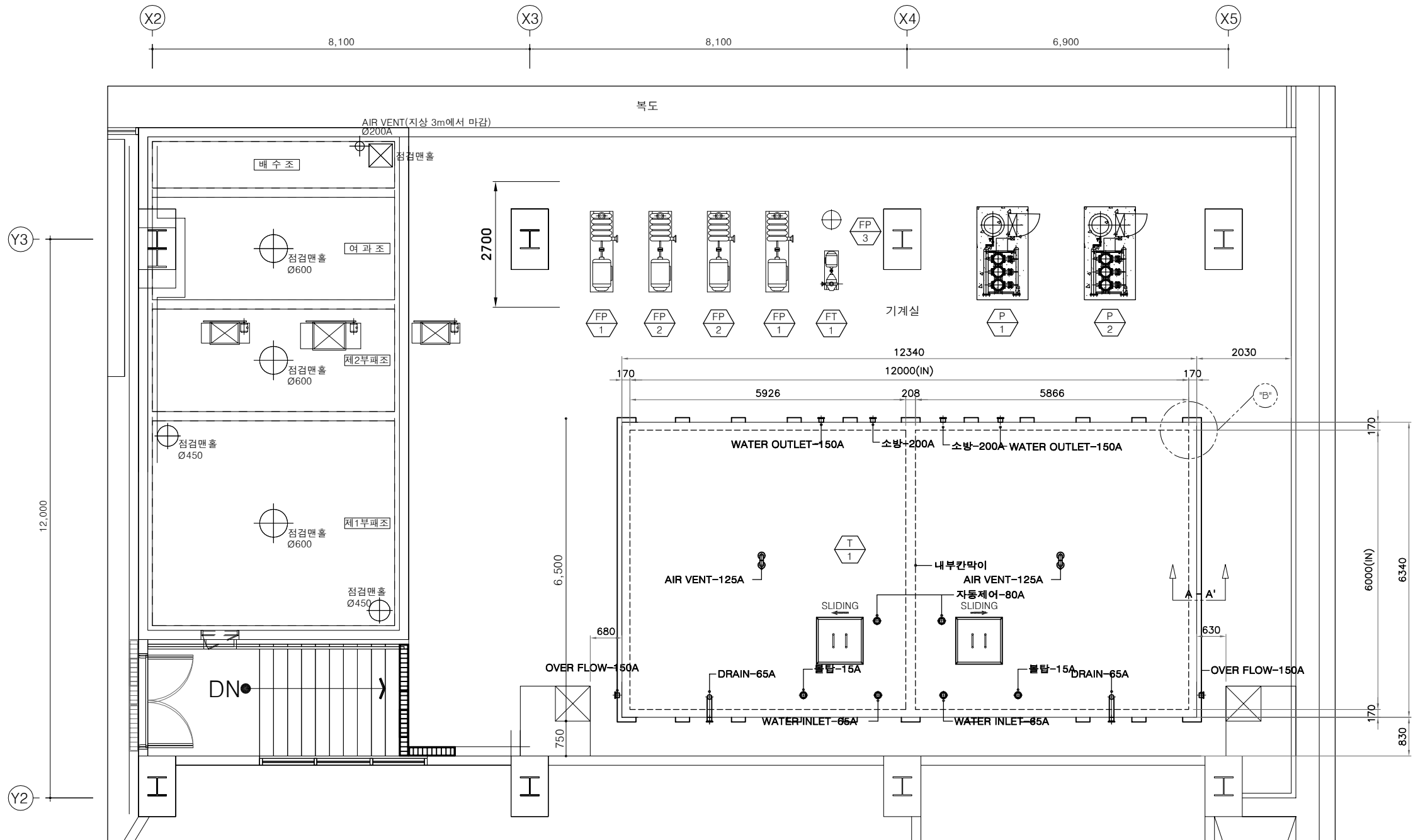
저수조 설치 평면도
