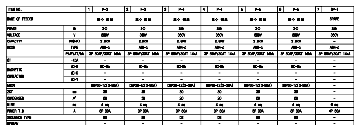
설치위치: B2F 펌프실
