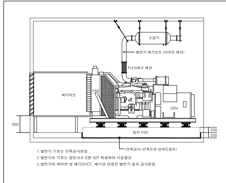
발전기설치 단면도
