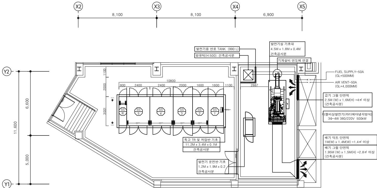
전기실 장비배치 평면도
