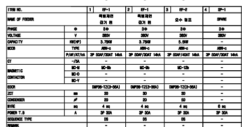
설치위치:PHF 기계실
