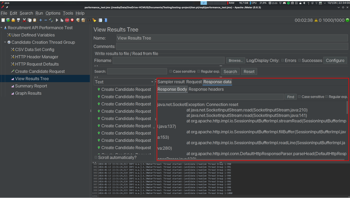
Hình 14: Các lỗi ghi nhận.
