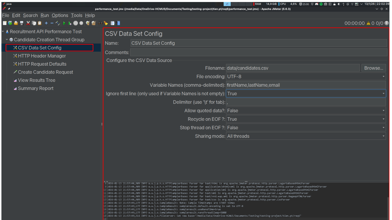
Hình 4: Cấu hình CSV Data Set Config để đọc dữ liệu từ file data/candidates.csv .
