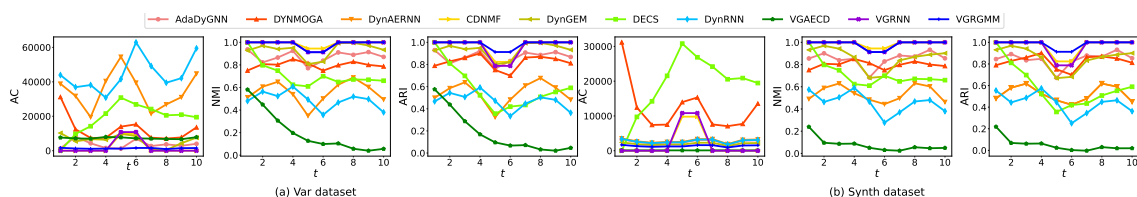
图 5-2 两种生成的动态网络的实验结果对比。(a) Var 数据集, (b) Synth 数据集。图中每个值是基于10次具有相同参数的随机生成网络的计算的平均值。
