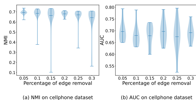
图 5-7 模型鲁棒性小提琴图
