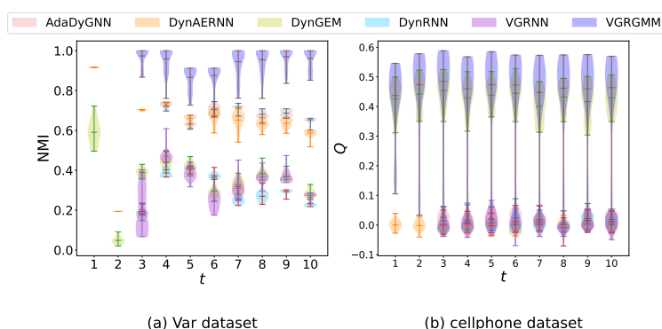
图 5-6 模型稳定性对比小提琴图
