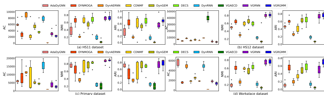
图 5-3 四个具有真相的真实世界动态网络的社团检测结果
