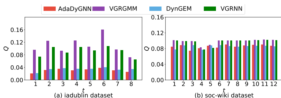
图 5-5 VGRGMM, AyaDyGNN, DynGEM和VGRGMM在大规模真实世界数据中的结果
