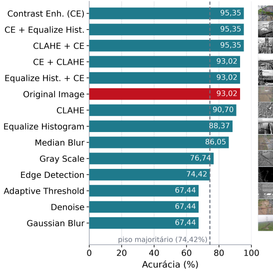
Fig. 4. Acurácia das estratégias de pré-processamento no dataset CPLID. A barra destacada é a imagem sem tratamento e a linha tracejada marca o piso majoritário. CE abrevia Contrast Enhancement .
