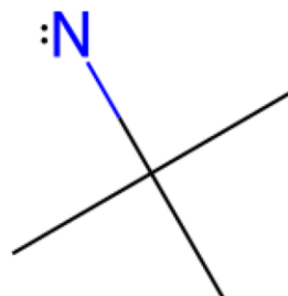
ligand764-0
