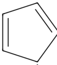
ligand22-0
