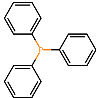
ligand28-0
