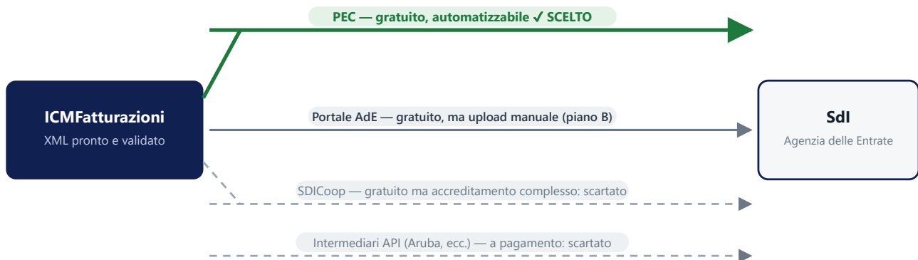
Fig. 2 — I quattro canali verso lo Sdl. La PEC unisce costo zero e automazione dall'applicativo.
