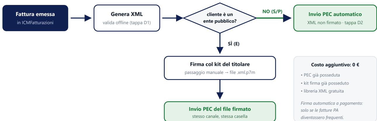
Fig. 3 — Flusso a regime per tipo di cliente: automatico per società e privati, un solo passaggio manuale per gli enti.
