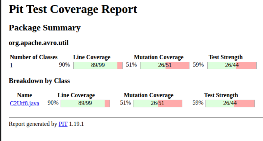
Figure 41: Report PIT della suite LLM Zero-Shot su C2Utf8.
