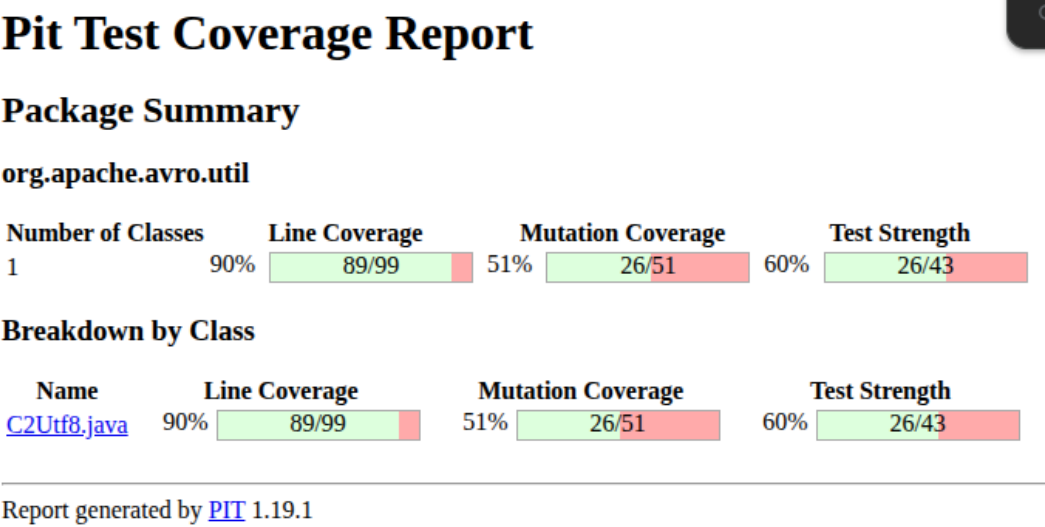
Figure 43: Report PIT della suite LLM ToT su C2Utf8.
