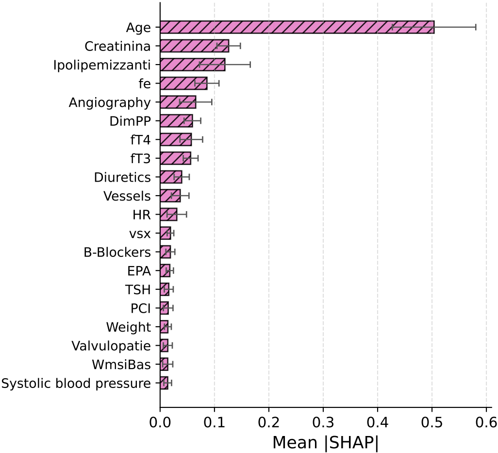
TabPFN - Cox
