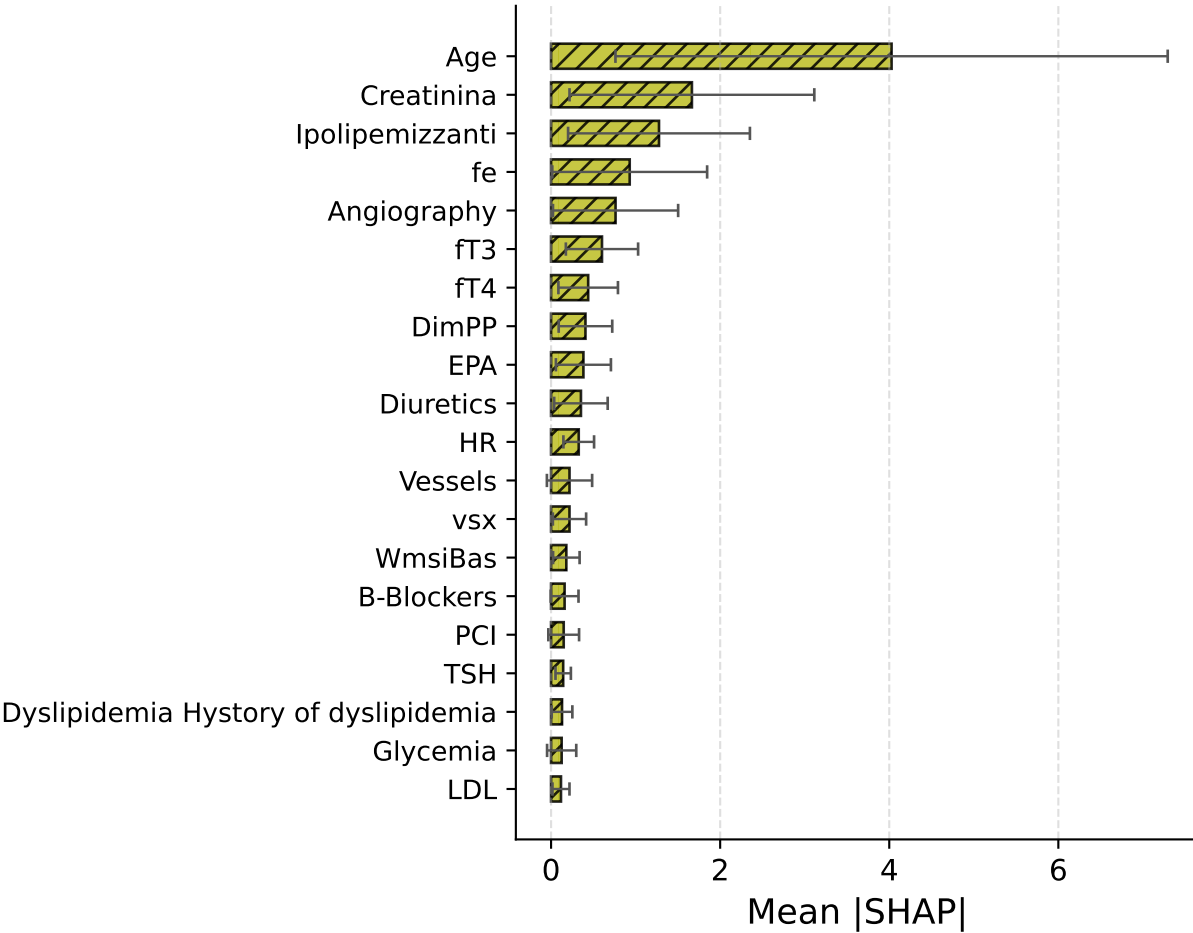
TabPFN - Cox
