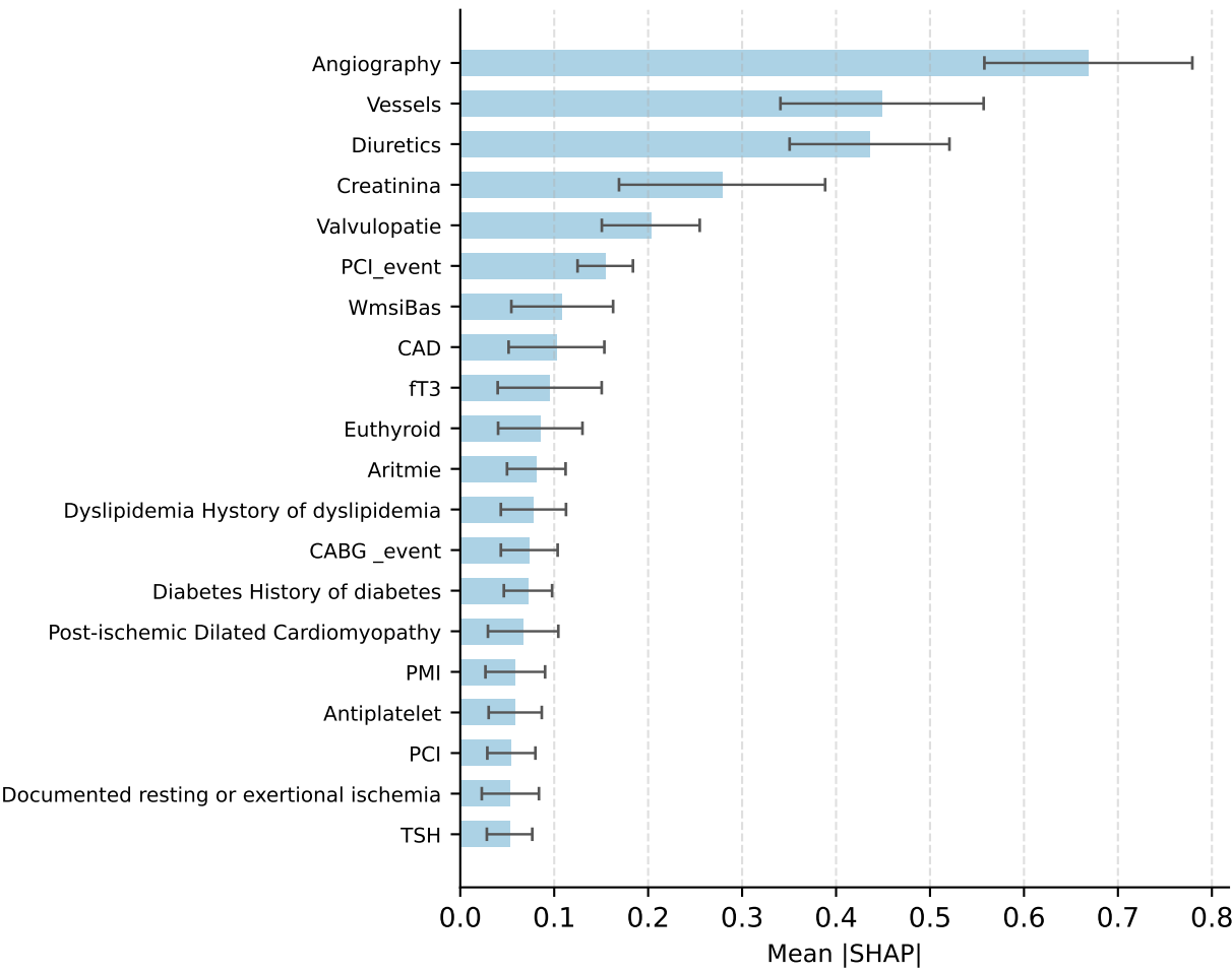
Cox
