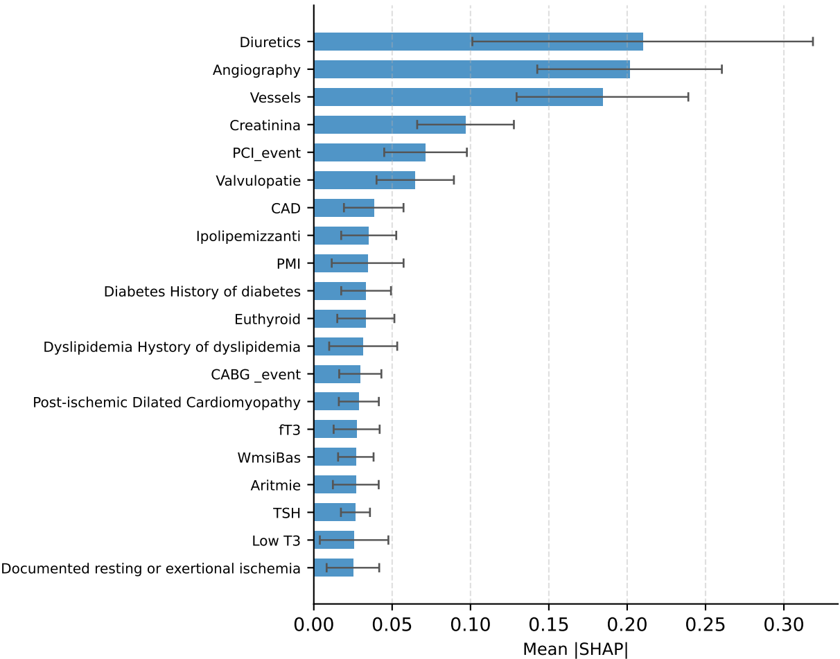
Cox
