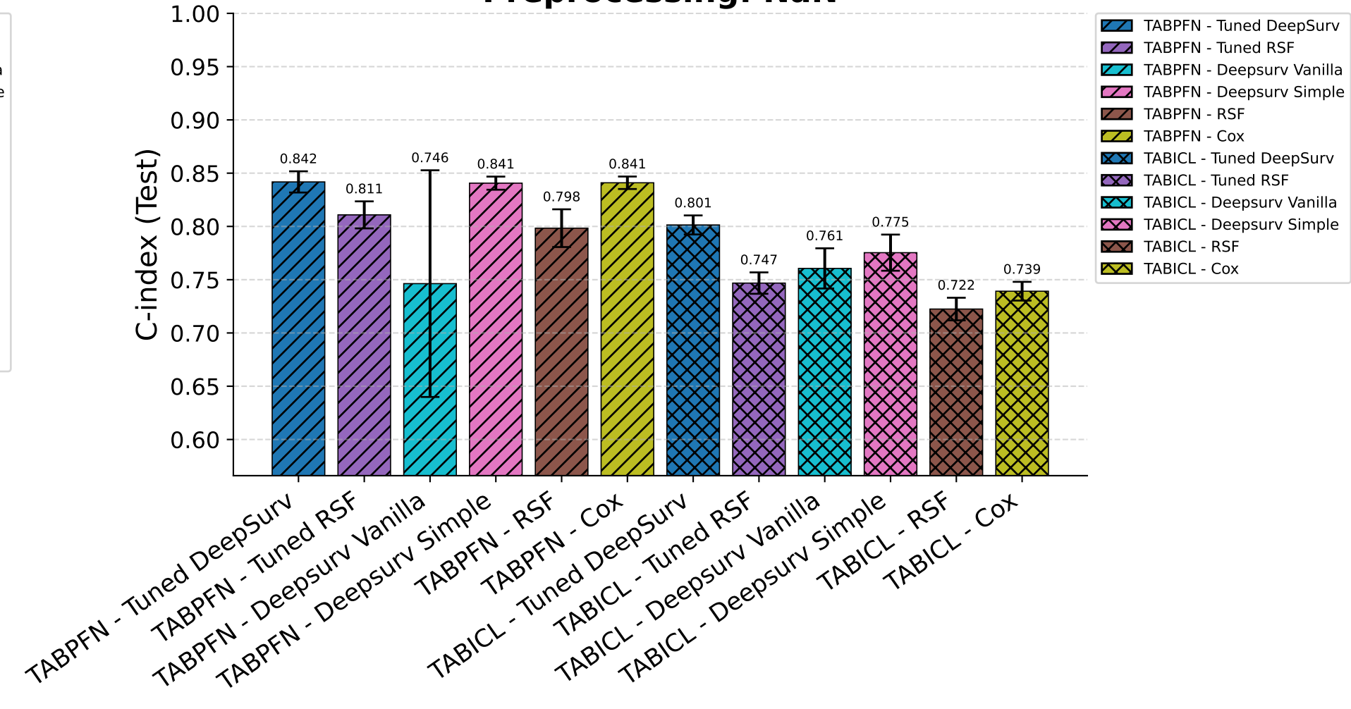
Preprocessing: NaN
