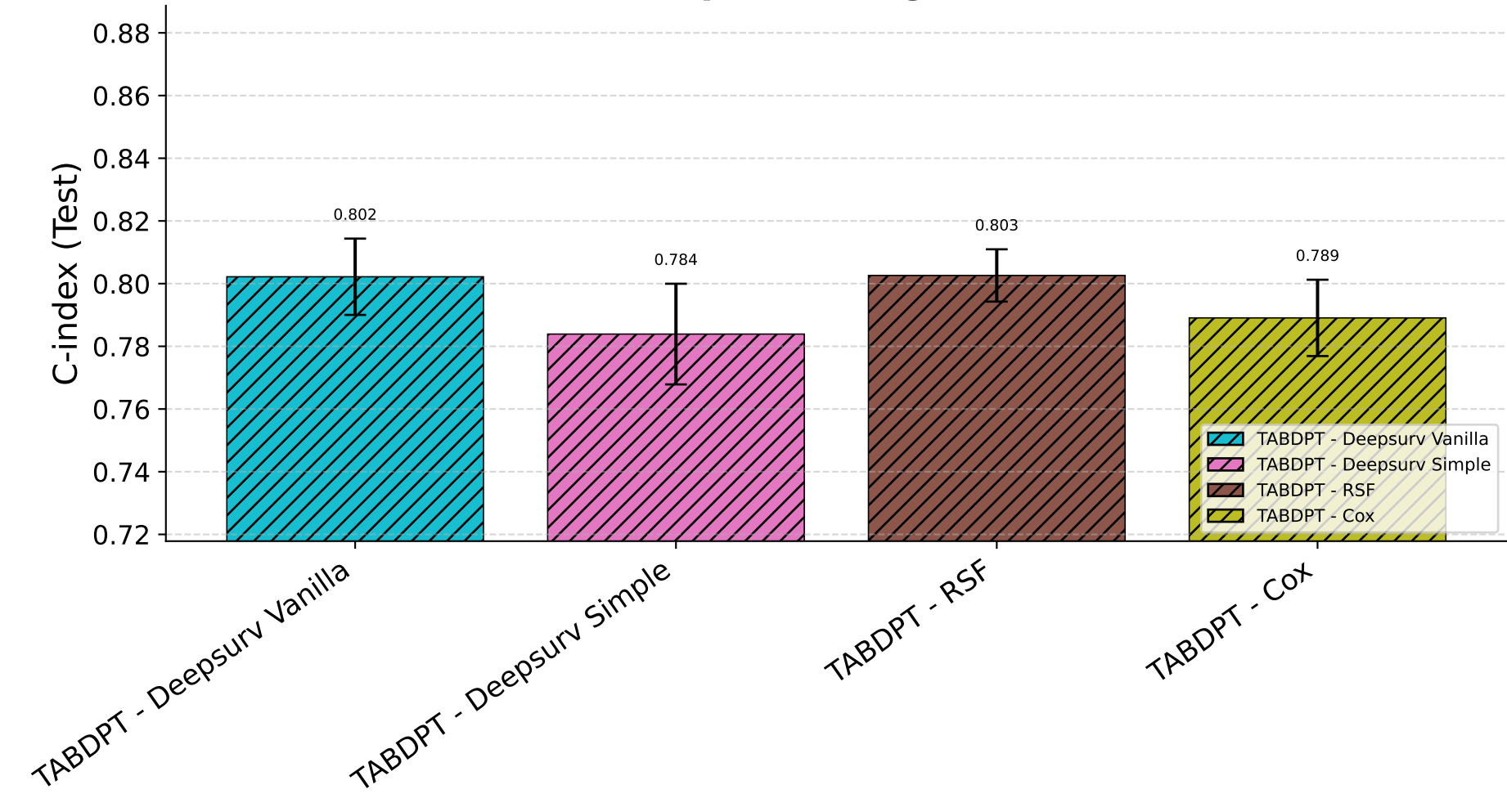
Preprocessing: NaN
