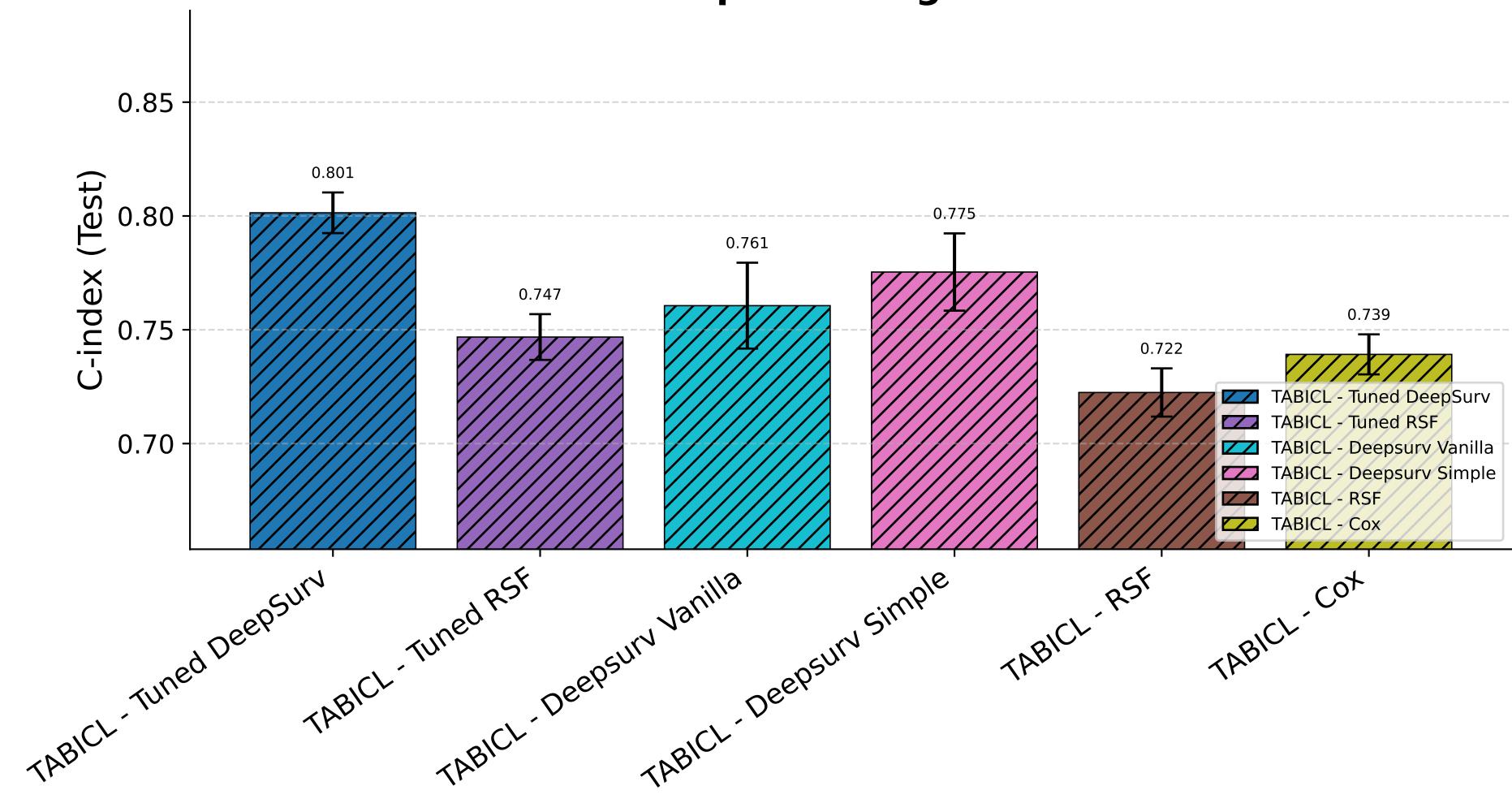
Preprocessing: NaN
