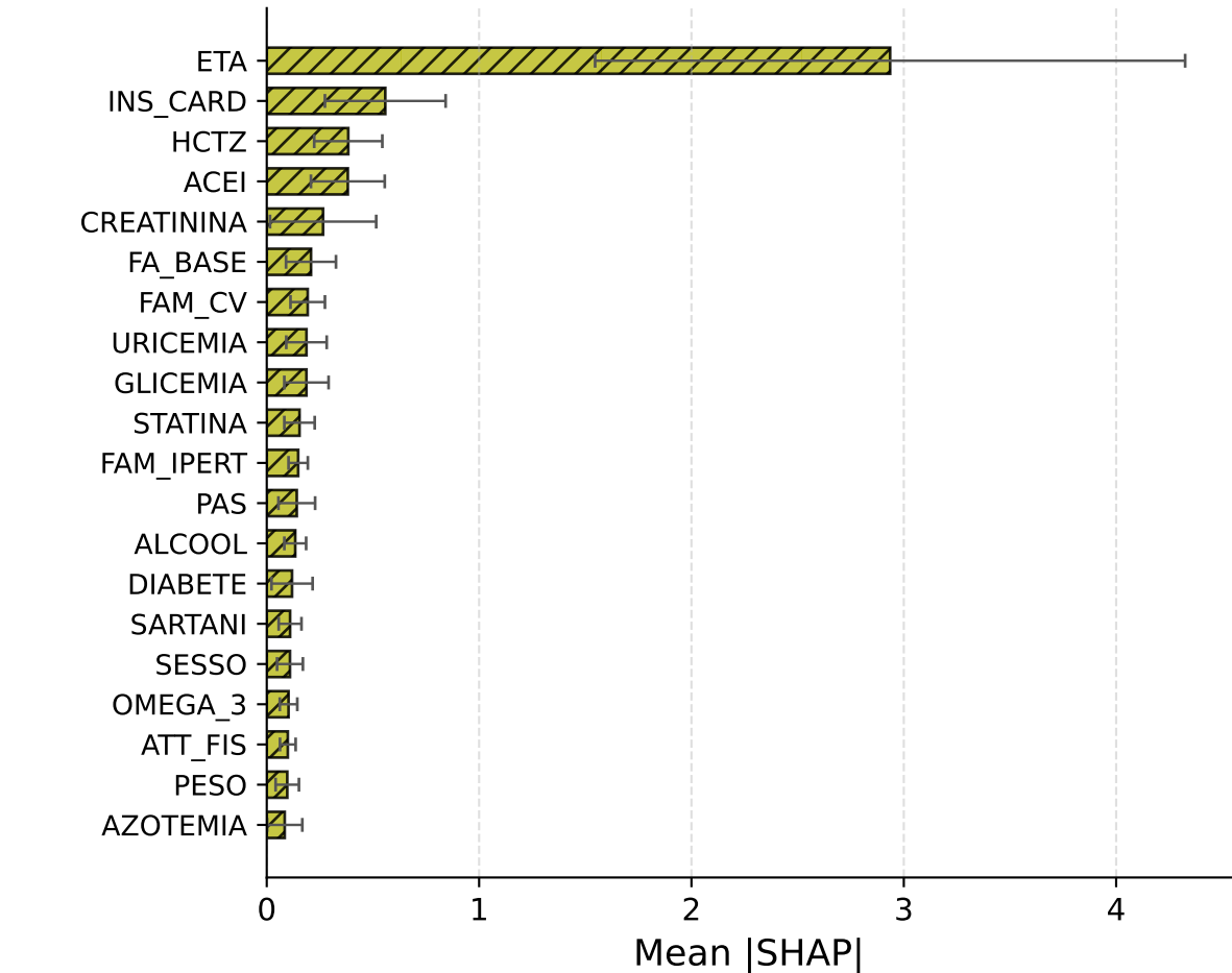
Cox
