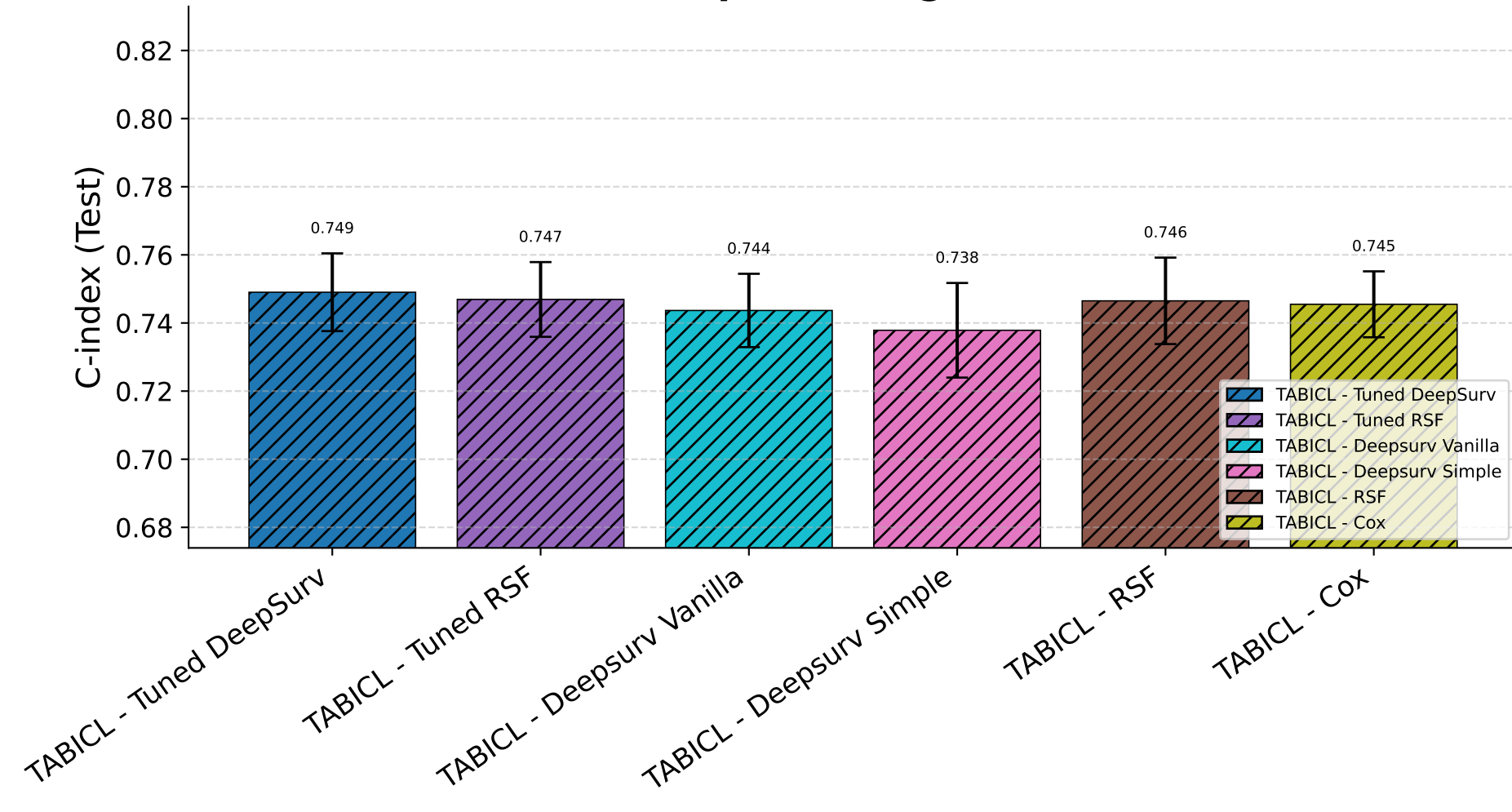
Preprocessing: NaN
