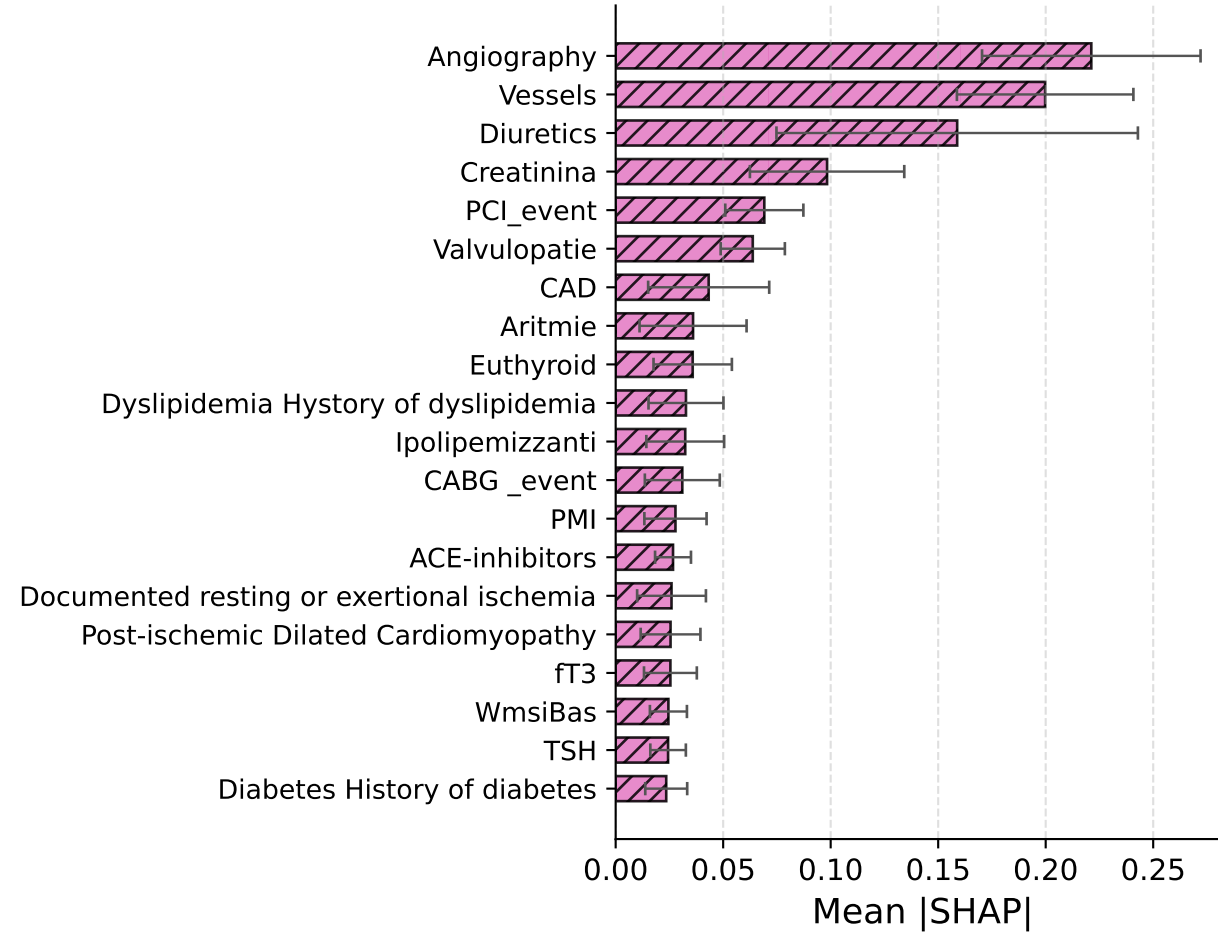
Cox
