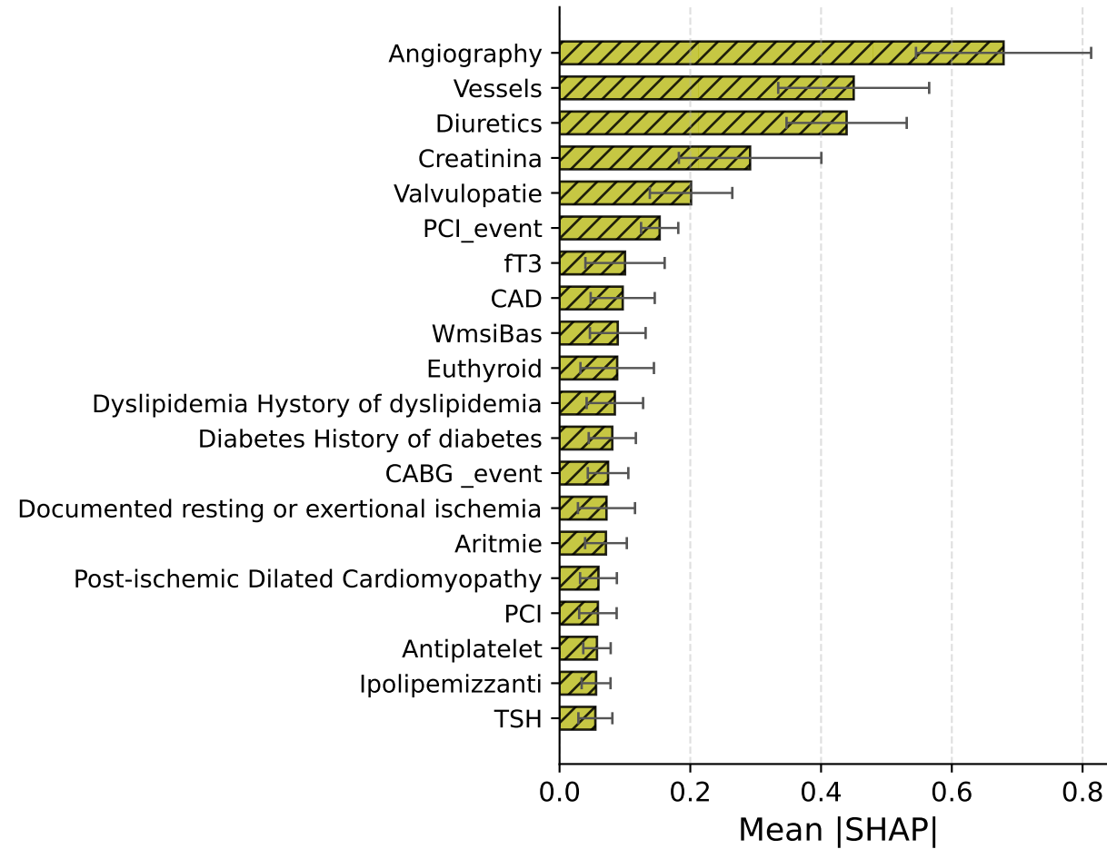
Cox
