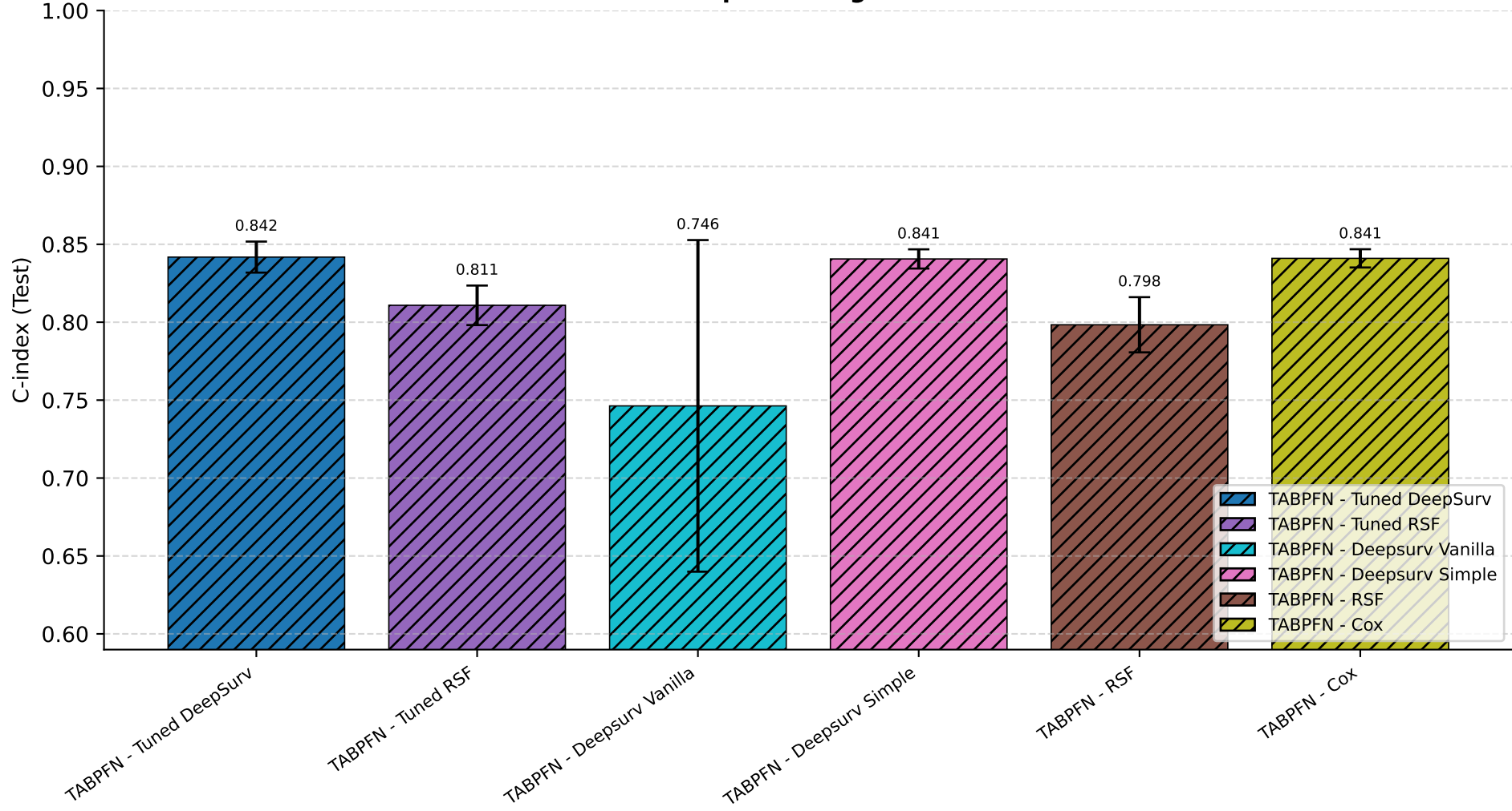
Preprocessing: NaN
