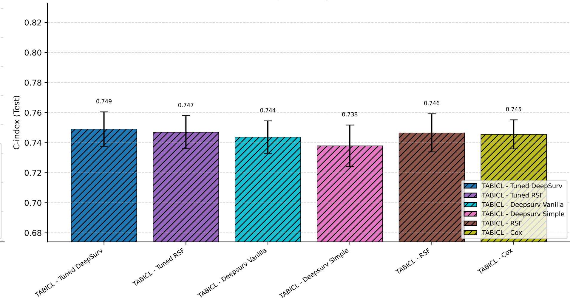
Preprocessing: NaN
