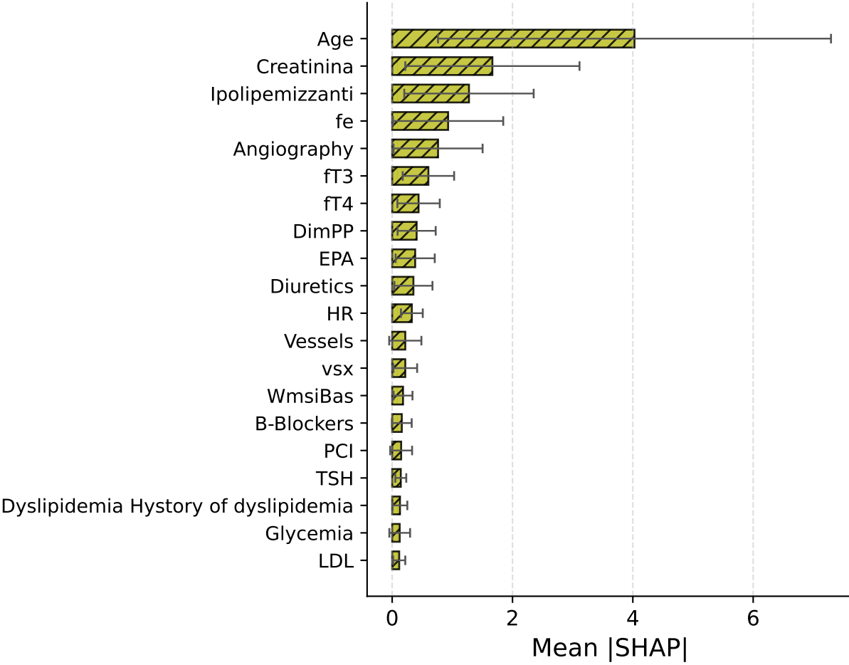
TabPFN - Cox
