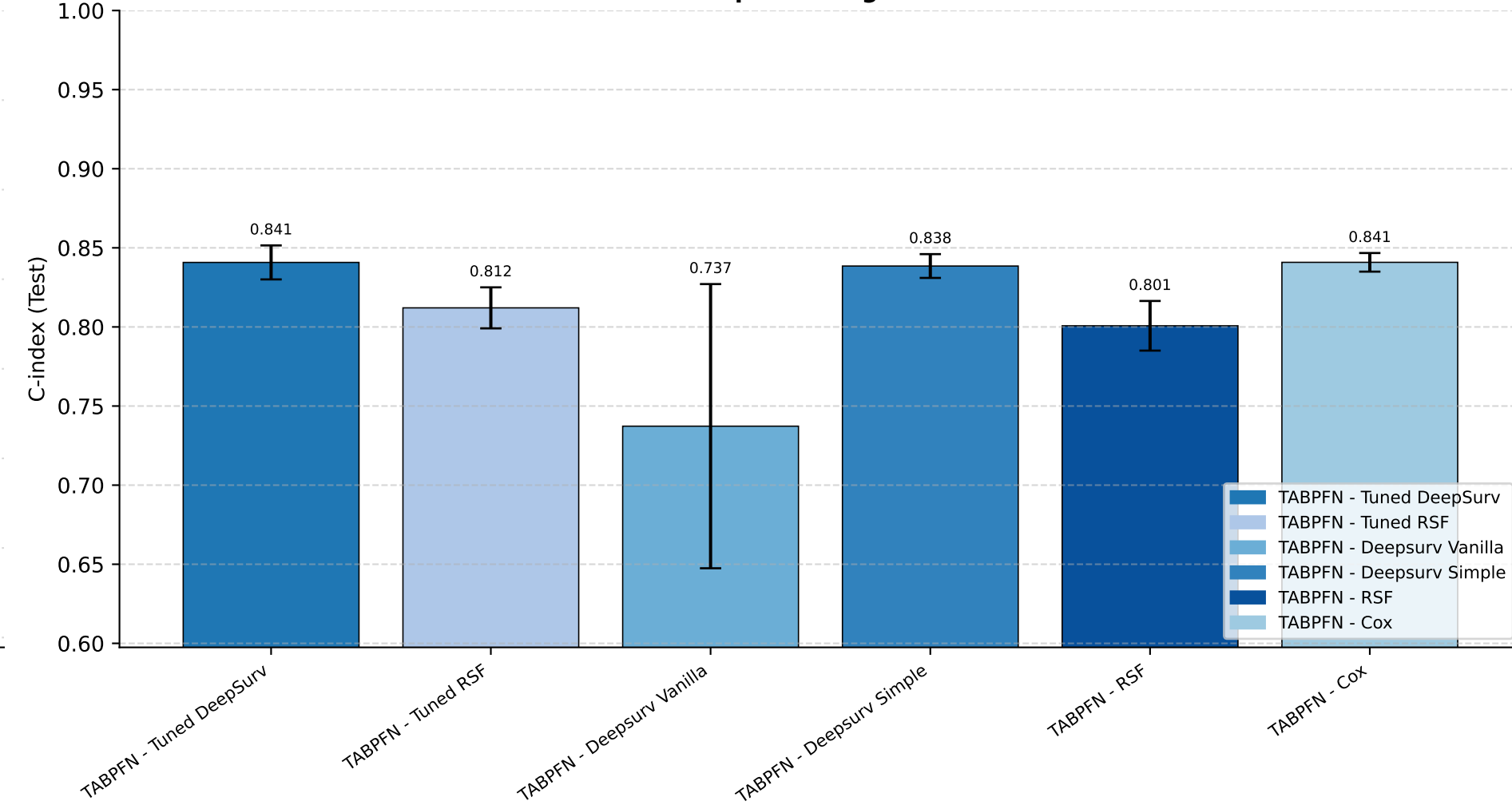
Preprocessing: NaN
