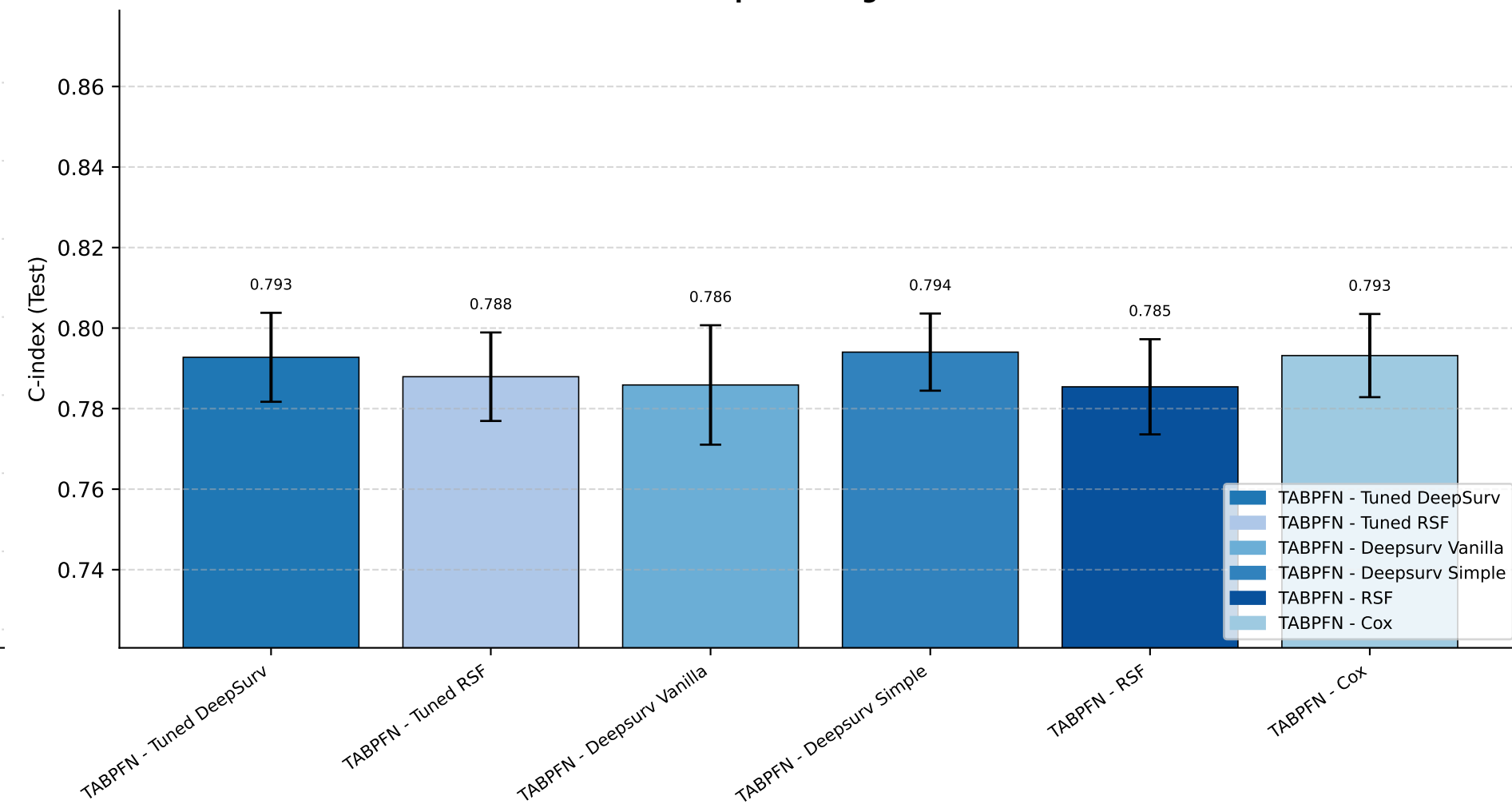
Preprocessing: NaN
