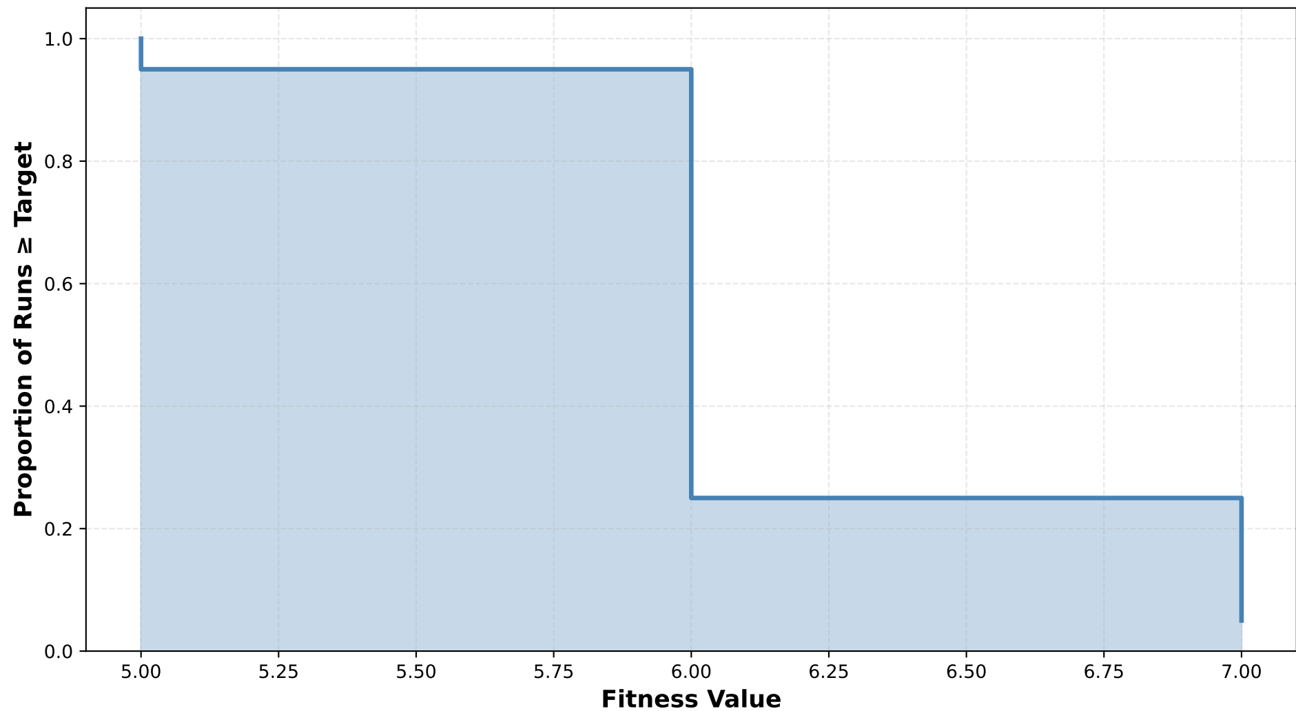
ECDF: F23 N-Queens (GA, D=49)
