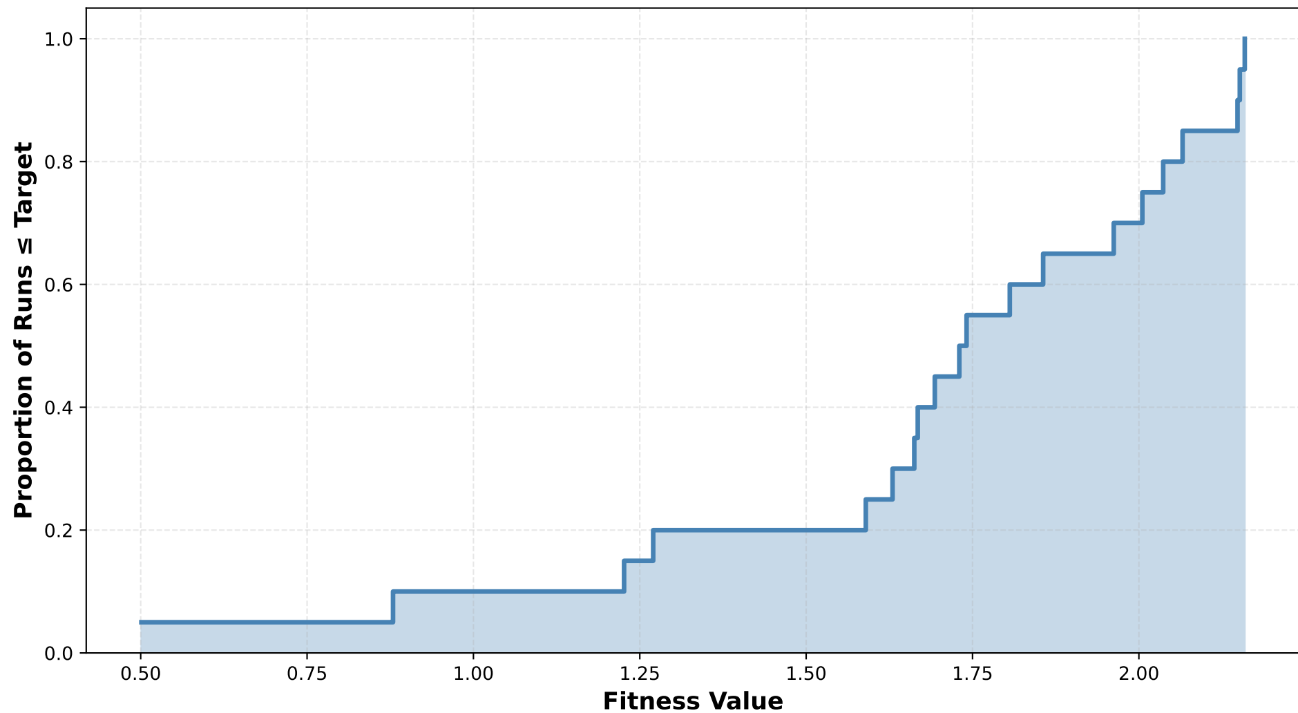
ECDF: F23 Katsuura (ES, D=10)
