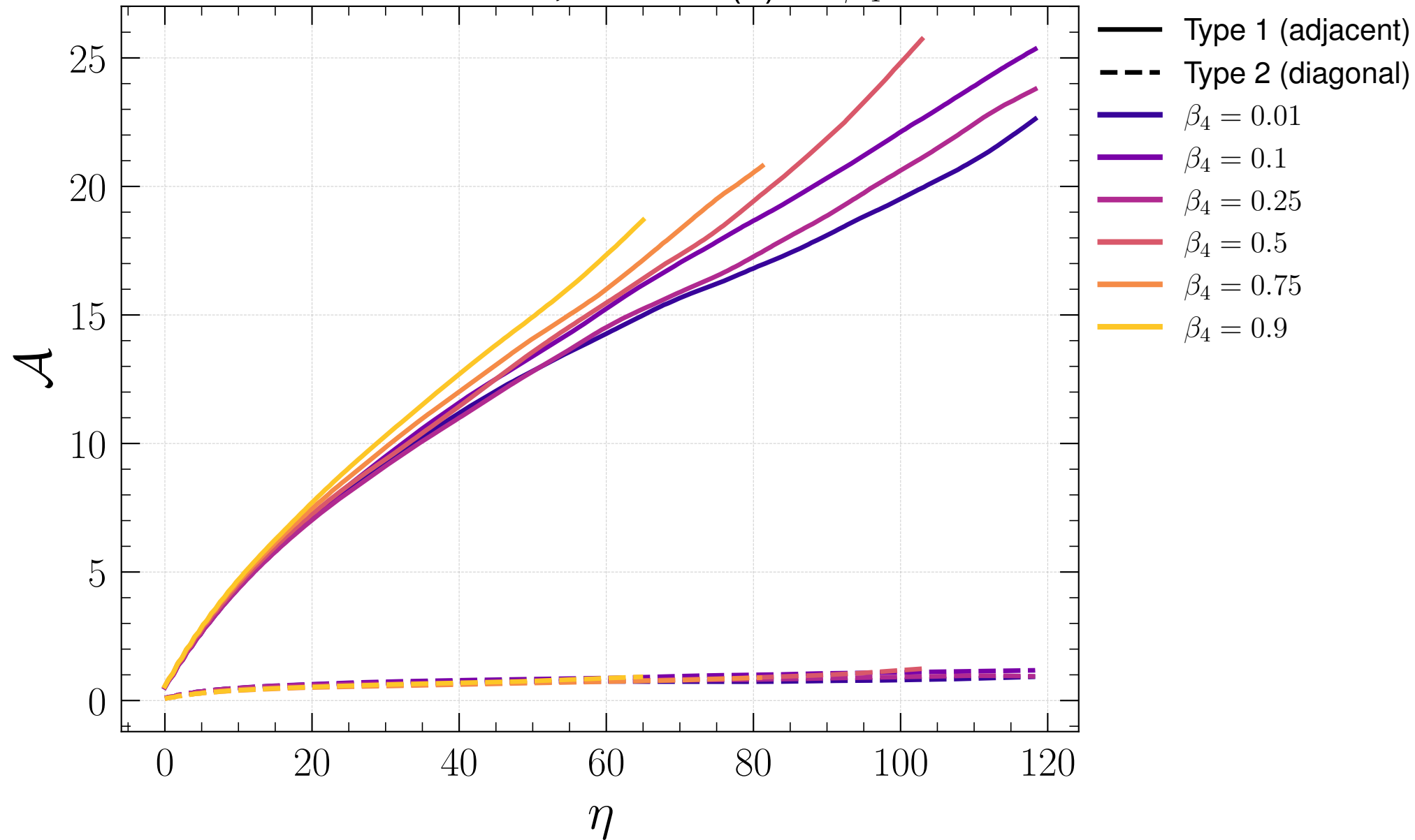
PRS Z4 wall area, Z4 \rightarrow U(1) as \beta_4 \rightarrow 0
