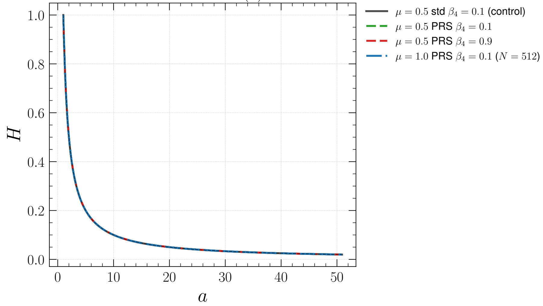
Hubble rate H(a)
