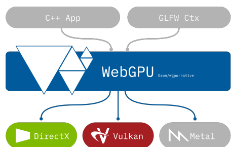
Figura 3.1: WebGPU Design
