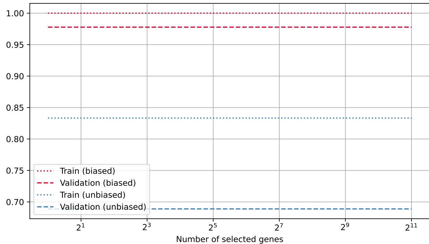
Lasso
