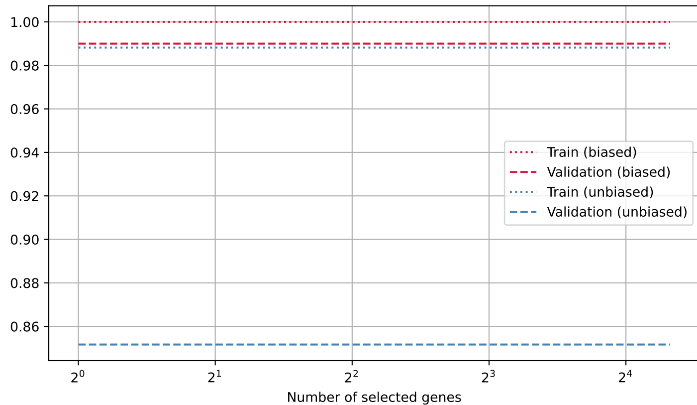
Lasso
