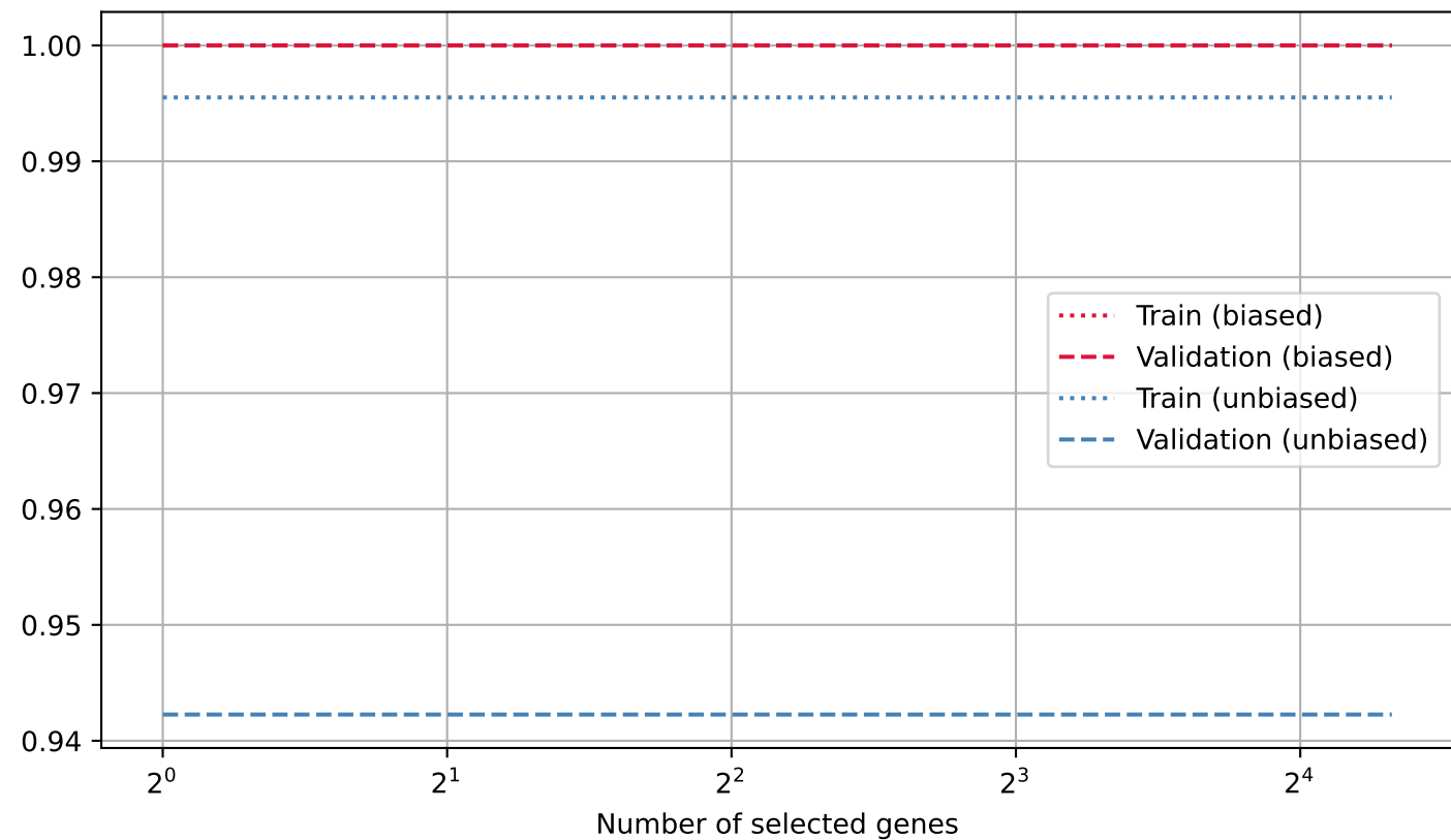
Lasso
