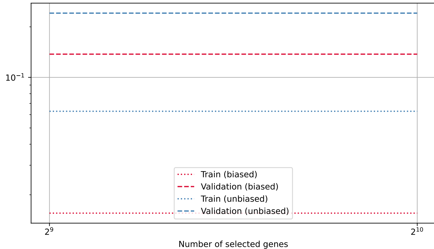
Lasso
