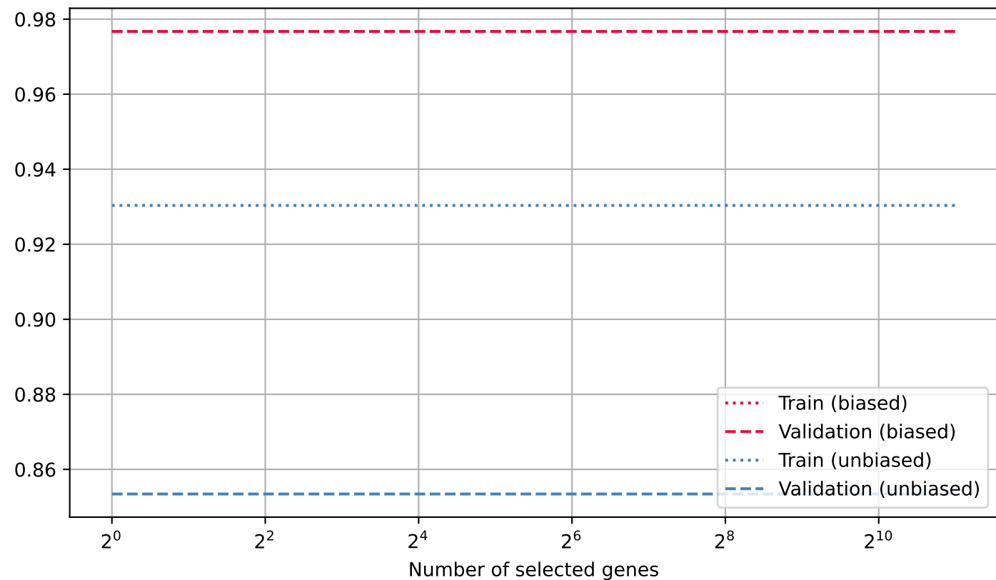
Lasso
