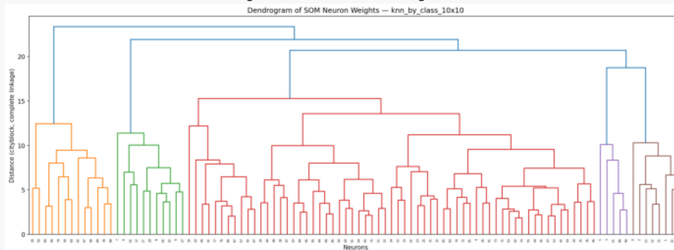
Dendrogram of SOM Neuron Weight Vectors
