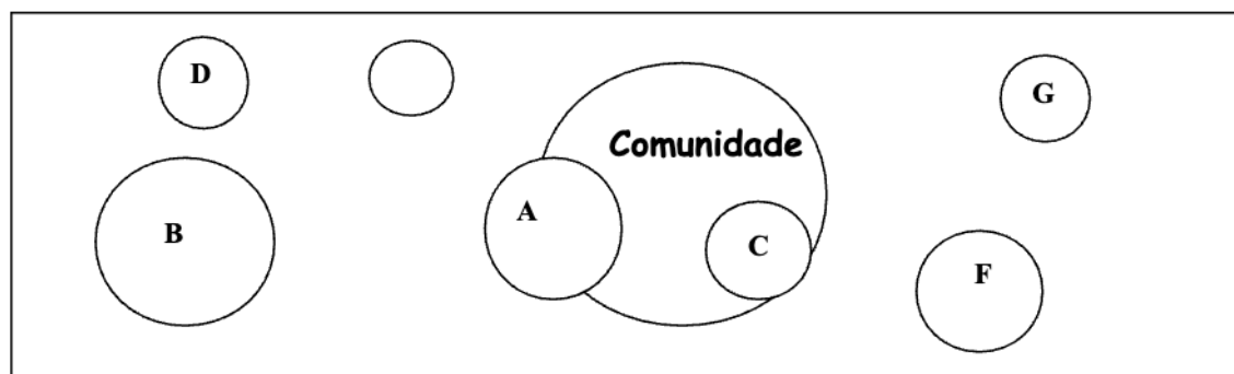
Diagrama de Venn
