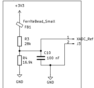
Voltaje Referencia XADC
