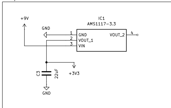
Voltaje Referencia 3.3V
