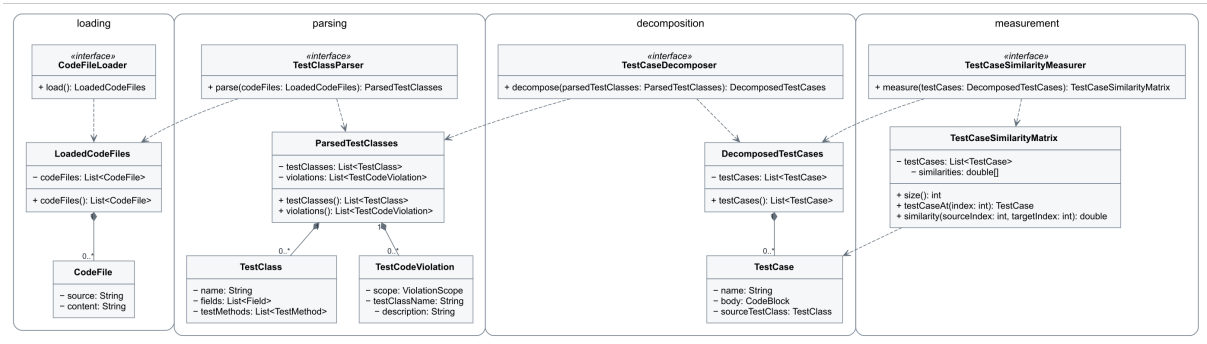
Figura 13 – Diagrama de classes do Róza até a etapa de medição
