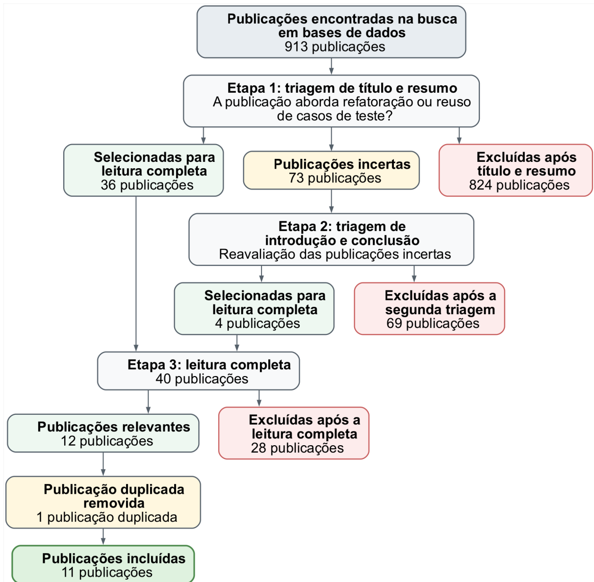
Figura 10 – Etapas de filtragem do estudo sistemático, da busca inicial até as 11 publicações incluídas
