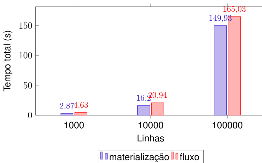
Figura 15 – Tempo total por modelo de execução em função do volume (multifonte): o sobrecusto do fluxo encolhe de +61% para +10% à medida que a escrita passa a dominar.
