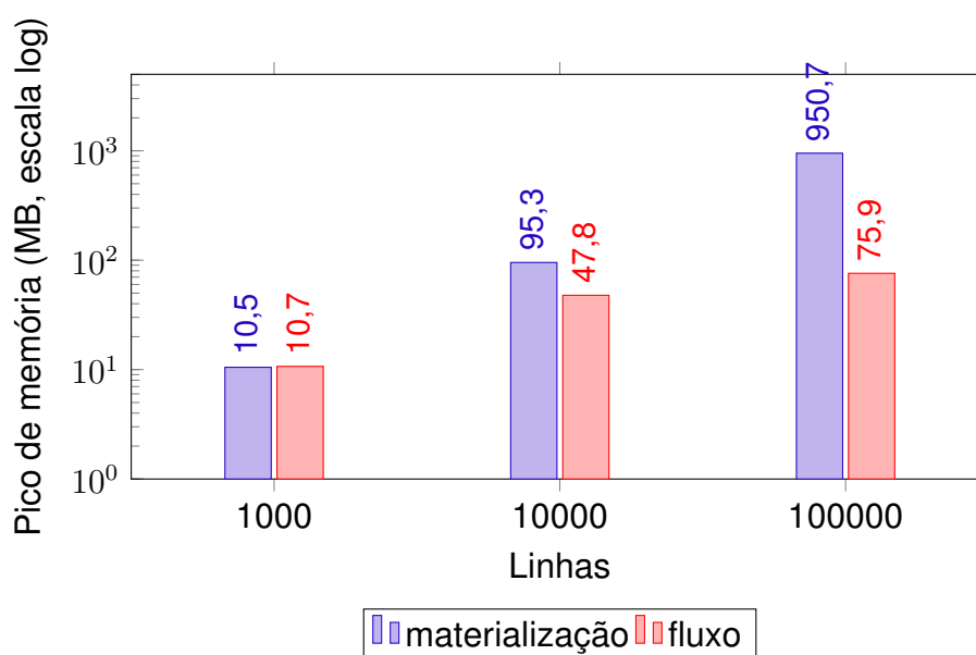
Figura 14 – Pico de memória por modelo de execução em função do volume (multifonte, escala logarítmica): a materialização cresce com o arquivo; o fluxo achata.
