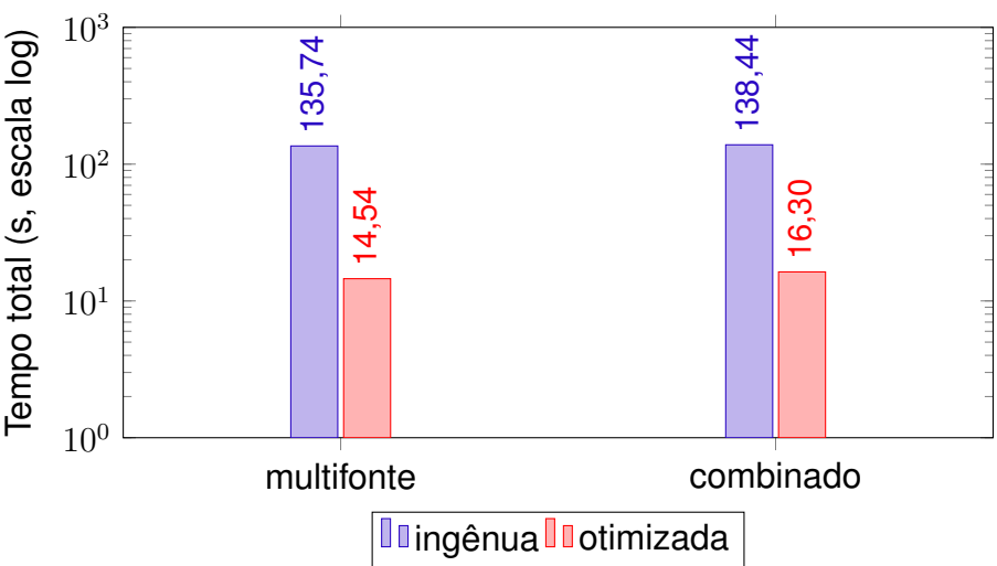
Figura 16 – Tempo total de importação por estratégia de escrita ( N = 10\,000 , materialização; eixo vertical em escala logarítmica). Campanha sem instrumentação de memória.
