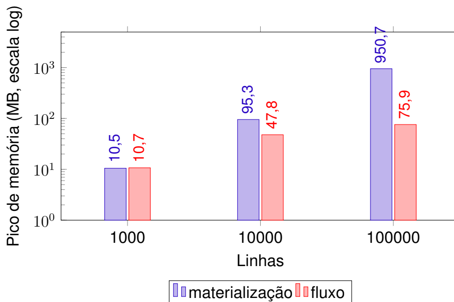
Figura 18 – Pico de memória por modelo de execução em função do volume (multifonte, escala logarítmica): a materialização cresce com o arquivo; o fluxo achata.
